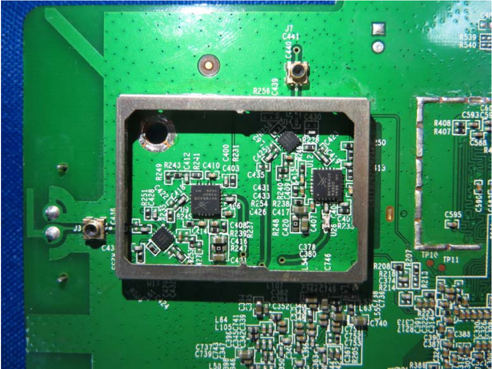
(12) EUT Photo (WCB6200Q)
