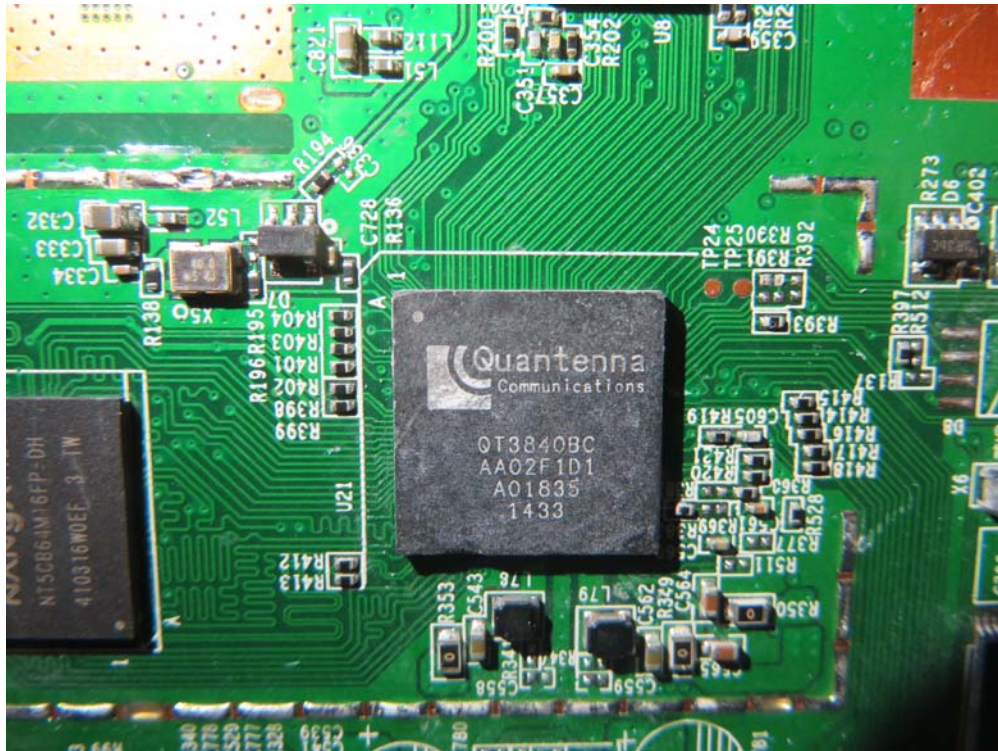
(19) EUT Photo (WCB6000Q)
