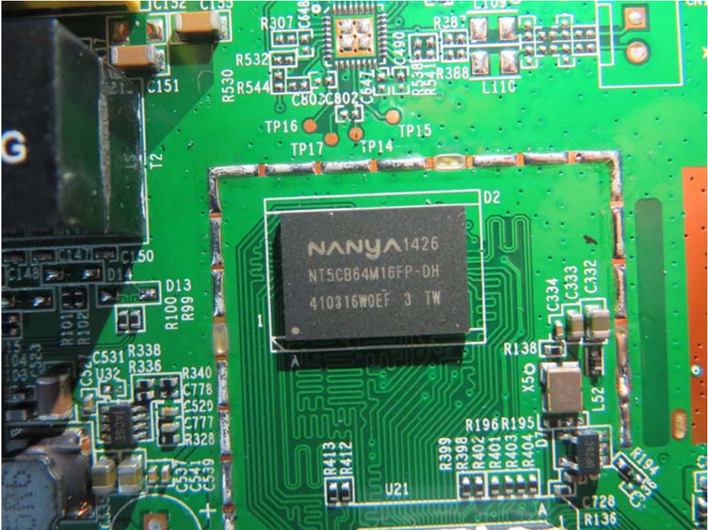
(8) EUT Photo (WCB6200Q)
