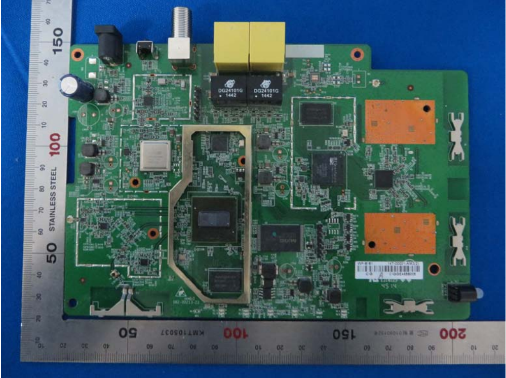
(5) EUT Photo (WCB6200Q)
