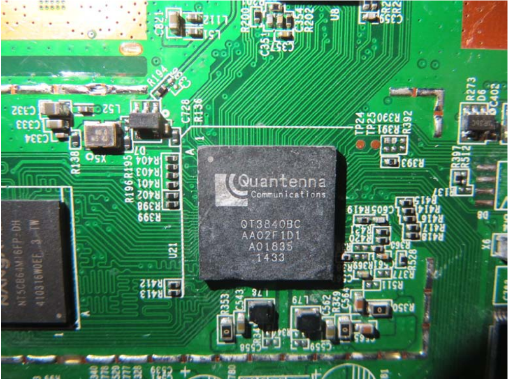
(6) EUT Photo (WCB6200Q)
