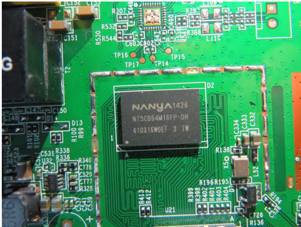
(20) EUT Photo (WCB6000Q)
