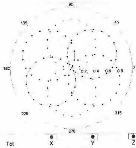
f=1800 MHz,R22
