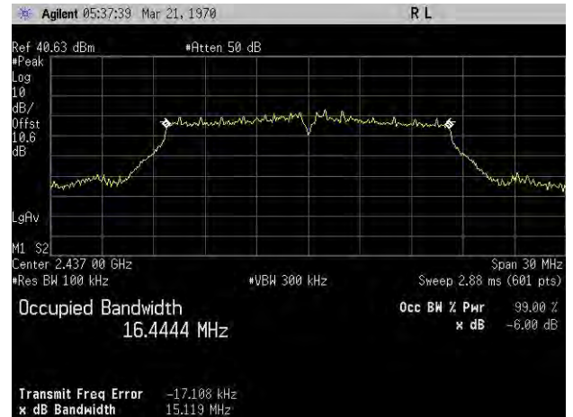
6 dB & 99 % EBW Chain 1
