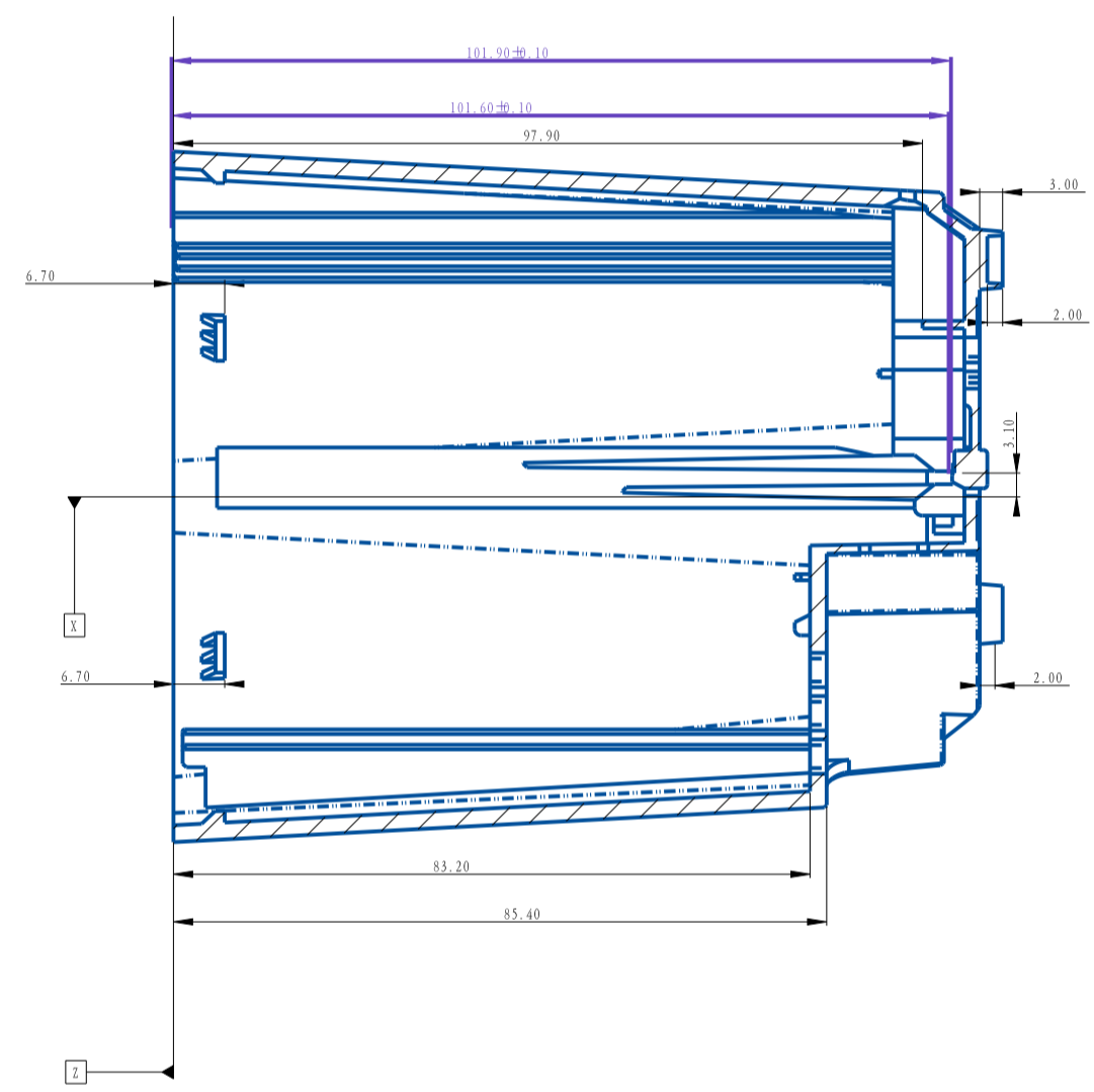
截面 B-B
