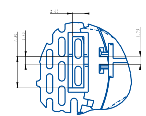
细节 B 比例 2:1
