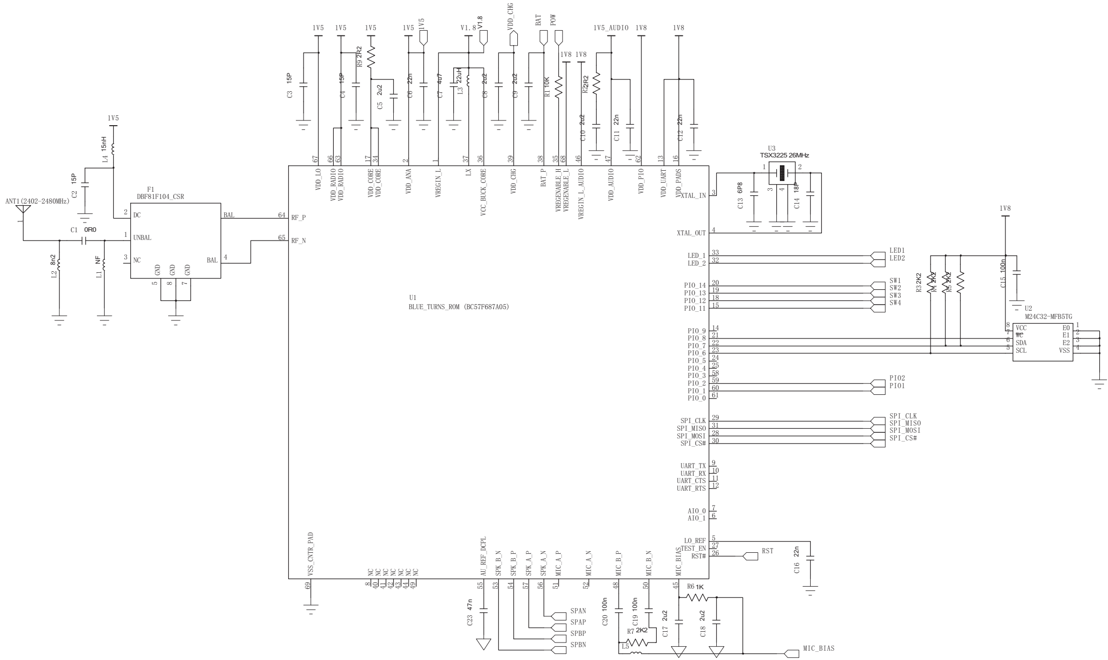
U7 BlueTooth Module
