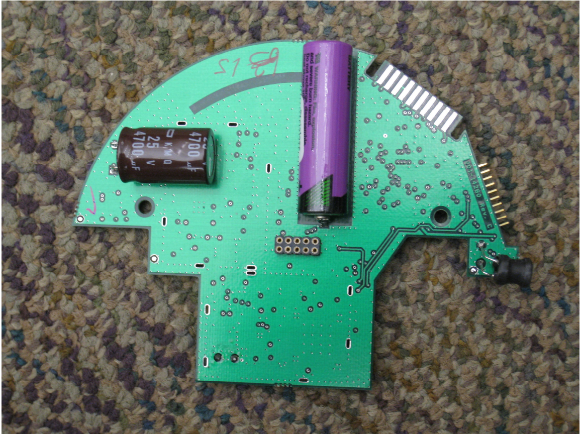
Bottom layer
