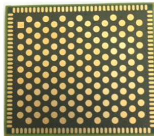
Fig. 2. LNADVW module bottom view
