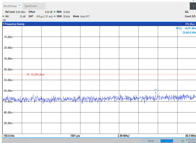
Band38-20MHz-QPSK-37850-1RB#0-Range2:0.15~30MHz
