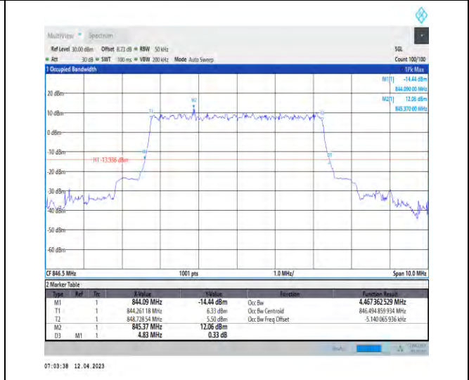
1-DC_2A_n5A-PC3-15-5+5-M+H-2-N/A-N/A-N/A-DF T-PI2BPSK-Outer_Full-25@0-Ant1-4.467-4.830-≤5-P ASS
