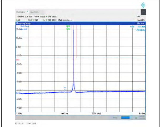
1-DC_5A_n2A-PC3-15-5+20-M+H-1-N/A-N/A-N/A-DF T-PI2BPSK-Inner_1RB_Left-1@1-1000-3000-2935.0 0--50.33--13-PASS
