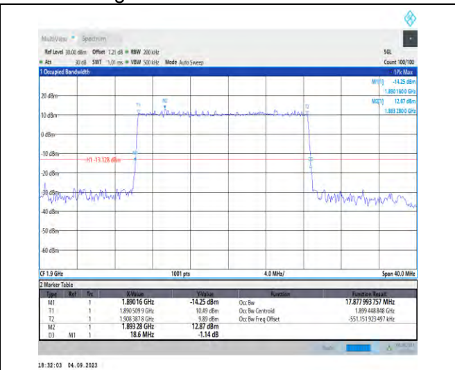
1-DC_5A_n2A-PC3-15-5+20-M+H-3-N/A-N/A-N/A-D FT-16QAM-Outer_Full-100@0-Ant1-17.848-22.520-≤ 20-PASS
