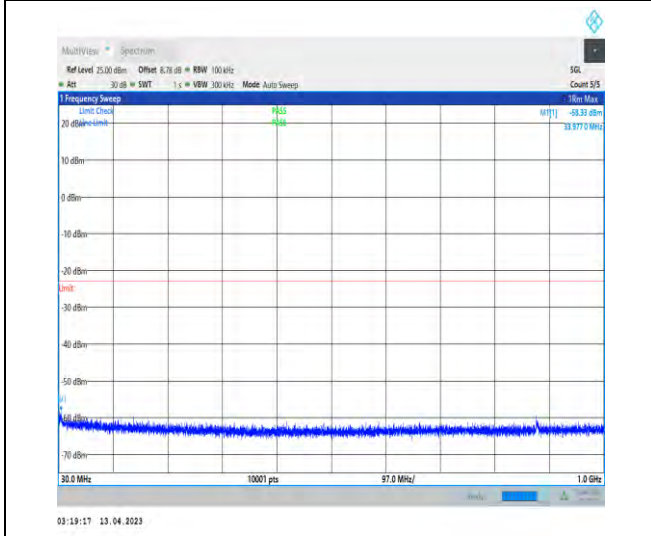
1-DC_5A_n2A-PC3-15-5+20-M+H-1-N/A-N/A-N/A-D FT-PI2BPSK-Inner_1RB_Left-1@1-30-1000-834.52- -58.33--23-PASS
