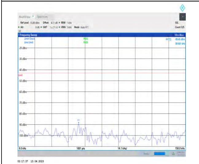
1-DC_5A_n2A-PC3-15-5+20-M+M-1-N/A-N/A-N/A-D FT-PI2BPSK-Inner_1RB_Left-1@1-0.009-0.15-0.06- -89.45--43-PASS
