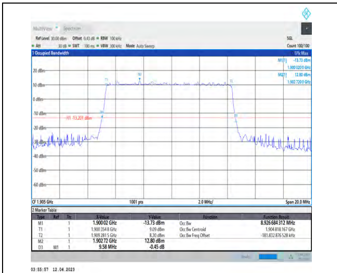
1-DC_5A_n2A-PC3-15-5+10-M+H-4-N/A-N/A-N/A-D FT-64QAM-Outer_Full-50@0-Ant1-8.927-9.580-≤10-PASS
