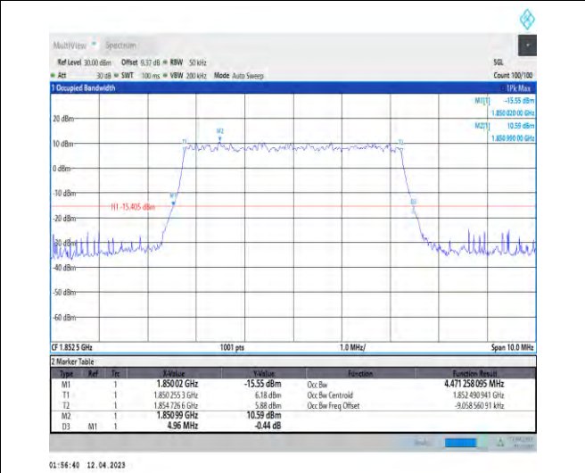
1-DC_5A_n2A-PC3-15-5+5-M+L-8-N/A-N/A-N/A-CP-64QAM-Outer_Full-25@0-Ant1-4.471-4.960-≤5-PAS S
