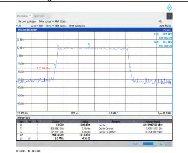
1-DC_5A_n2A-PC3-15-5+10-M+H-5-N/A-N/A-N/A-D FT-256QAM-Outer_Full-50@0-Ant1-8.92-9.600-≤10-PASS
