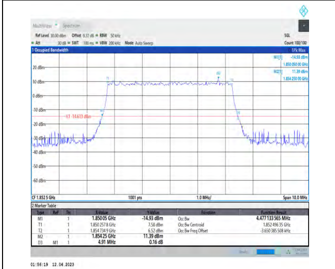
1-DC_5A_n2A-PC3-15-5+5-M+L-7-N/A-N/A-N/A-CP-16QAM-Outer_Full-25@0-Ant1-4.477-4.910-≤5-PAS S
