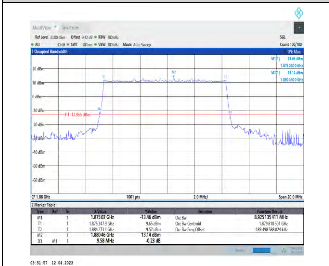
1-DC_5A_n2A-PC3-15-5+10-M+M-3-N/A-N/A-N/A-D FT-16QAM-Outer_Full-50@0-Ant1-8.925-9.580-≤10-PASS
