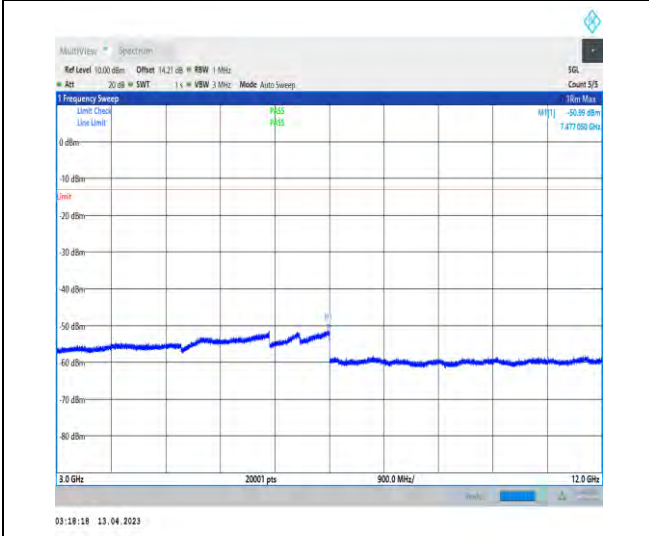
1-DC_5A_n2A-PC3-15-5+20-M+M-1-N/A-N/A-N/A-D FT-PI2BPSK-Inner_1RB_Left-1@1-3000-12000-744 7.80--50.99--13-PASS
