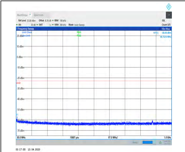
1-DC_5A_n2A-PC3-15-5+20-M+M-1-N/A-N/A-N/A-D FT-PI2BPSK-Inner_1RB_Left-1@1-30-1000-834.52- -58.44--23-PASS
