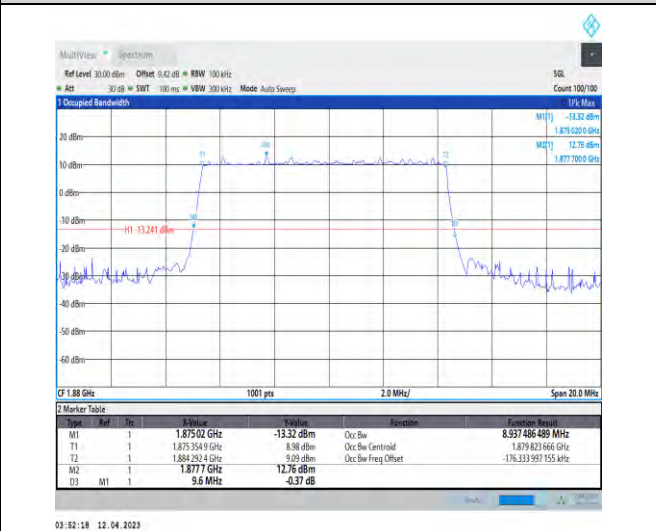
1-DC_5A_n2A-PC3-15-5+10-M+M-4-N/A-N/A-N/A-D FT-64QAM-Outer_Full-50@0-Ant1-8.937-9.600-≤10-PASS
