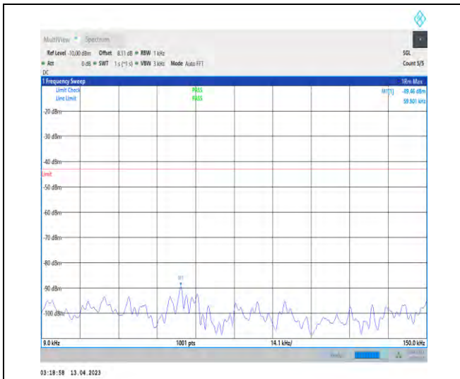
1-DC_5A_n2A-PC3-15-5+20-M+H-1-N/A-N/A-N/A-D FT-PI2BPSK-Inner_1RB_Left-1@1-0.009-0.15-0.06- -89.46--43-PASS
