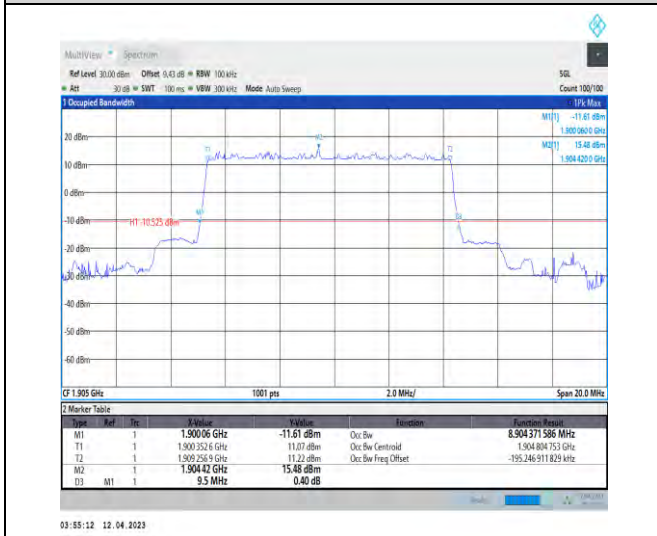
1-DC_5A_n2A-PC3-15-5+10-M+H-2-N/A-N/A-N/A-D FT-PI2BPSK-Outer_Full-50@0-Ant1-8.904-9.500≤10-PASS
