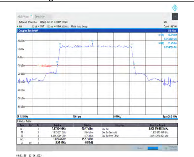
1-DC_5A_n2A-PC3-15-5+10-M+M-2-N/A-N/A-N/A-D FT-PI2BPSK-Outer_Full-50@0-Ant1-8.907-9.540-≤10-PASS
