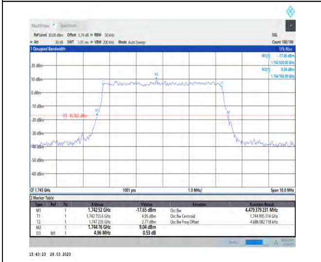
1-N66-15-5-M-6-CP-QPSK-Outer_Full-25@0-Ant1-4. 479-4.960-≤5-PASS
