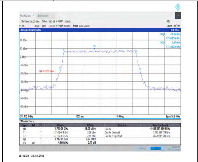
1-N66-15-5-L-6-CP-QPSK-Outer_Full-25@0-Ant1-4. 49-4.960-≤5-PASS
