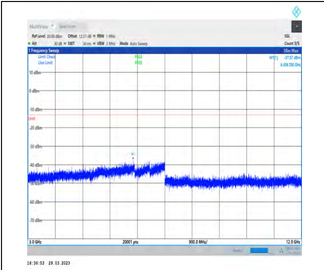
1-N66-15-40-H-1-DFT-PI2BPSK-Inner_1RB_Left-1 @1-3000-12000-Ant1-6458.25--37.57--13-PASS
