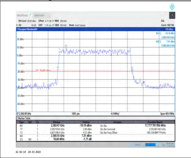
1-N41-30-20-M-5-DFT-256QAM-Outer_Full-50@0-A nt1-17.778-18.840-≤20-PASS
