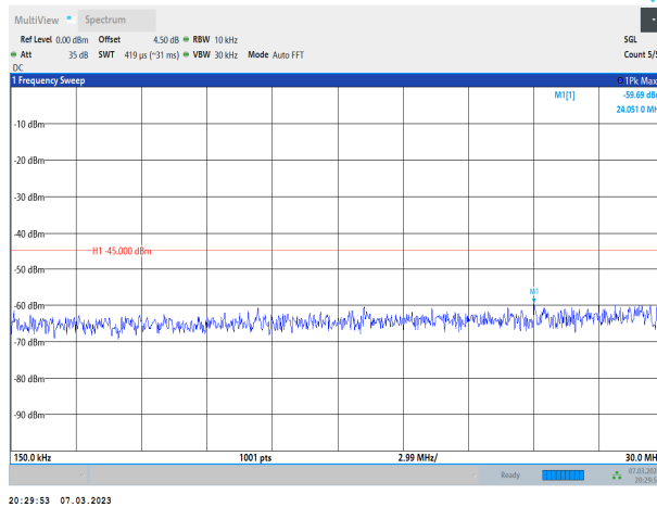
Band41-20MHz-QPSK-39750-1RB#0-Range2:0.15~30MHz
