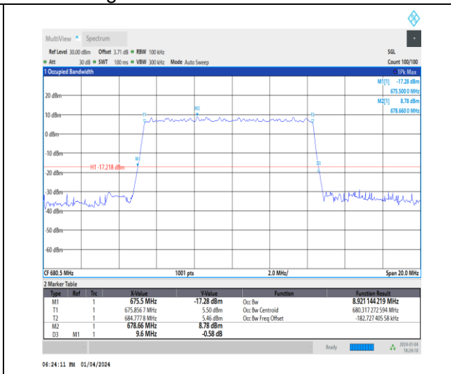
1-N71-15-10-M-5-DFT-256QAM-Outer_Full-50@0-A nt1-8.921-9.600-≤10-PASS
