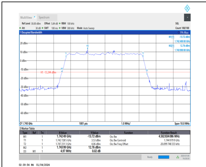
1-N66-15-5-M-9-CP-256QAM-Outer_Full-25@0-Ant1 -4.503-4.970-≤5-PASS
