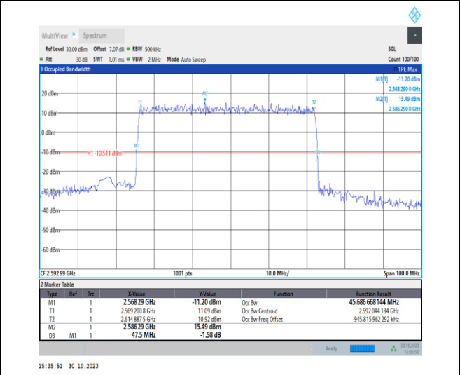
1-N41-30-50-M-1-DFT-QPSK-Outer_Full-128@0-Ant 1-45.687-47.500-≤50-PASS
