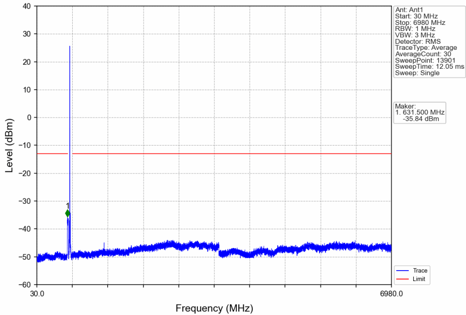
Band71_20MHz_QPSK_MCH_683MHz_RB_1_0_NTNV
