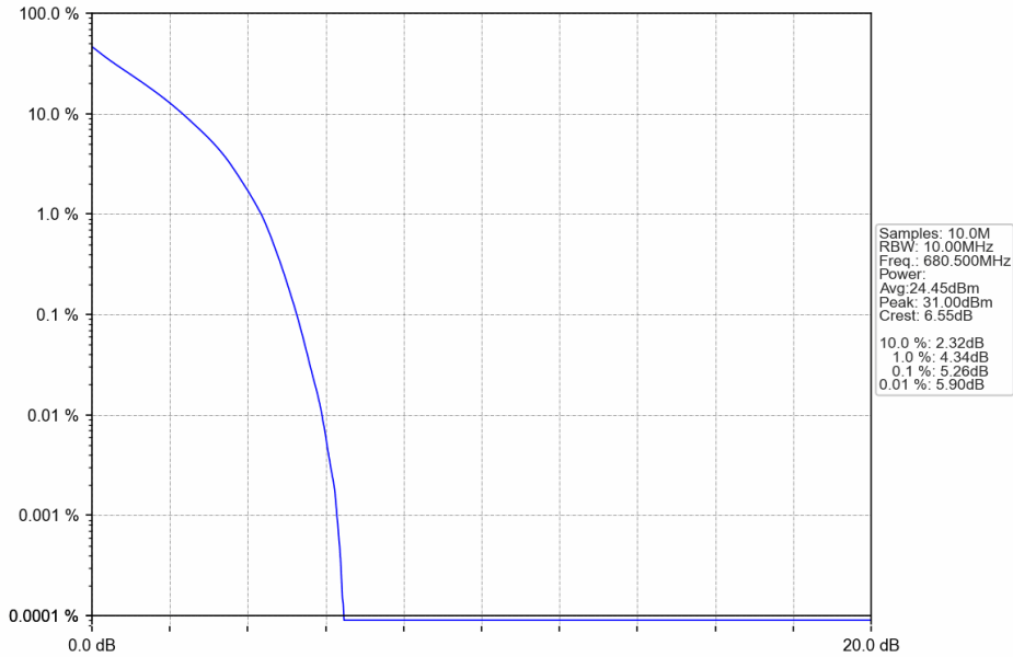
Band71_10MHz_QPSK_MCH_680.5MHz_RB_50_0_NTNV
