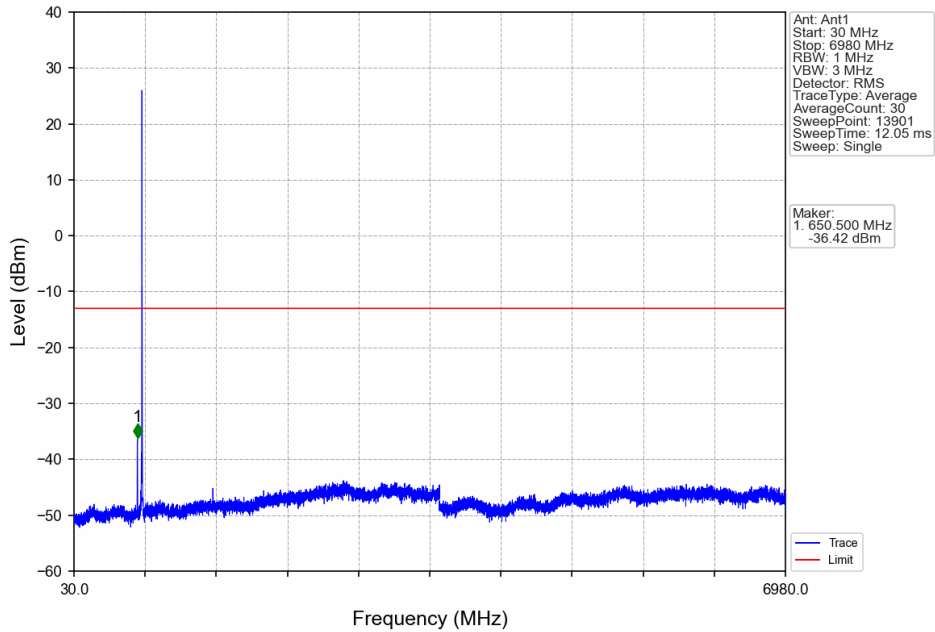
Band71_5MHz_QPSK_HCH_695.5MHz_RB_1_0_NTNV
