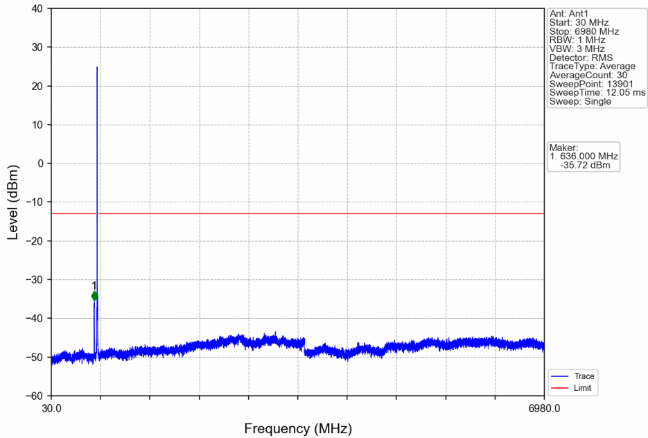
Band71_10MHz_QPSK_MCH_680.5MHz_RB_1_0_NTNV
