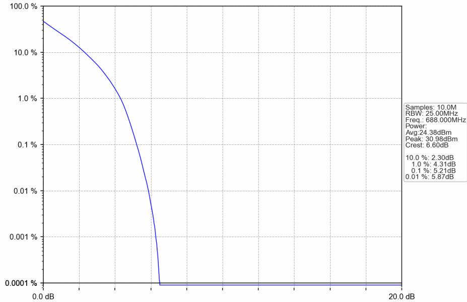
Band71_20MHz_QPSK_HCH_688MHz_RB_100_0_NTNV
