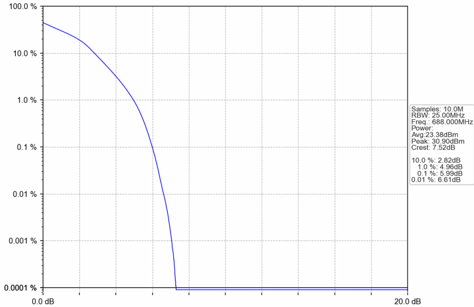
Band71_20MHz_16QAM_HCH_688MHz_RB_100_0_NTNV
