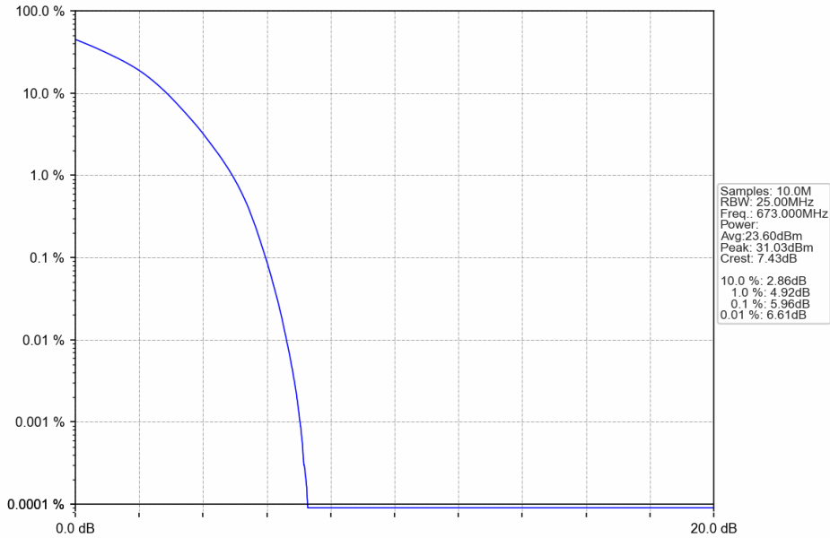
Band71_20MHz_16QAM_LCH_673MHz_RB_100_0_NTNV
