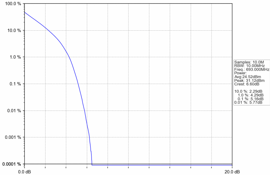
Band71_10MHz_QPSK_HCH_693MHz_RB_50_0_NTNV
