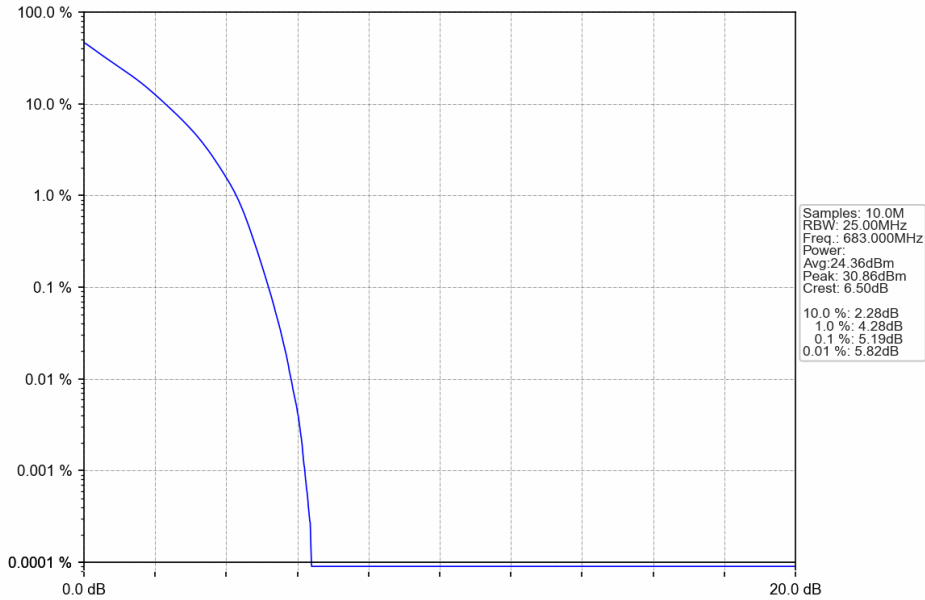
Band71_20MHz_QPSK_MCH_683MHz_RB_100_0_NTNV
