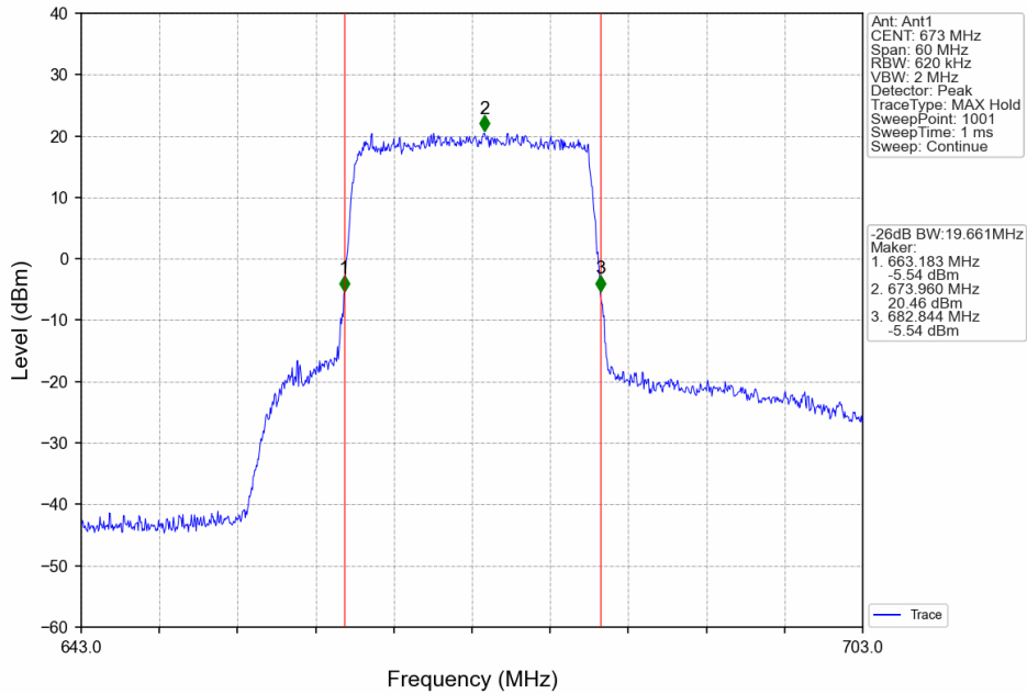
Band71_20MHz_16QAM_LCH_673MHz_RB_100_0_NTNV
