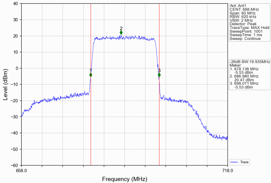
Band71_20MHz_16QAM_HCH_688MHz_RB_100_0_NTNV
