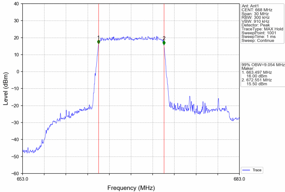
Band71_10MHz_QPSK_LCH_668MHz_RB_50_0_NTNV
