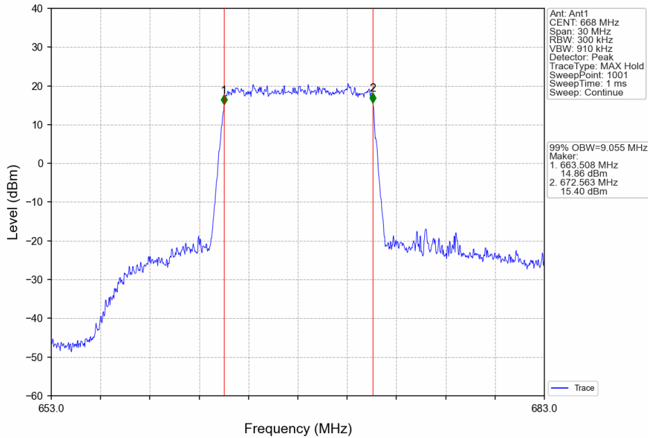
Band71_10MHz_16QAM_LCH_668MHz_RB_50_0_NTNV
