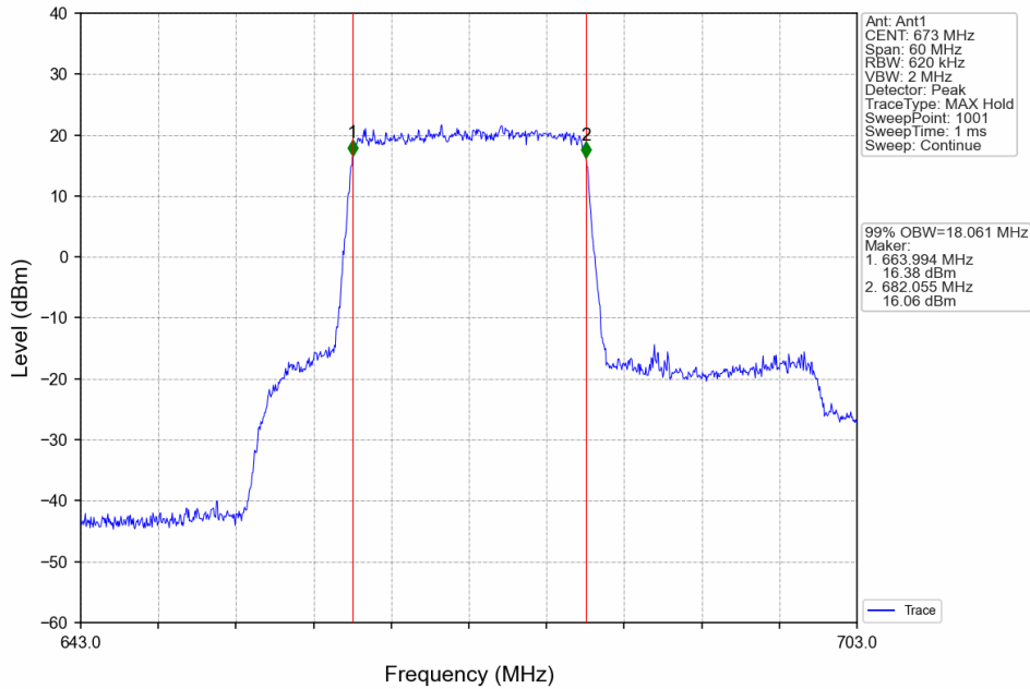
Band71_20MHz_QPSK_LCH_673MHz_RB_100_0_NTNV
