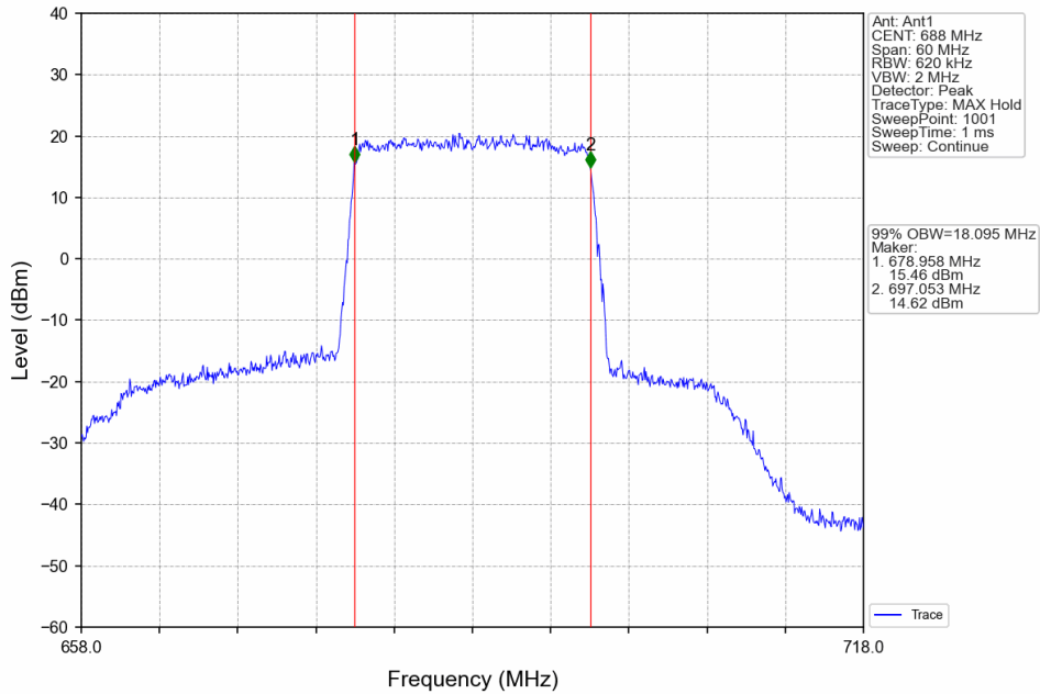
Band71_20MHz_16QAM_HCH_688MHz_RB_100_0_NTNV
