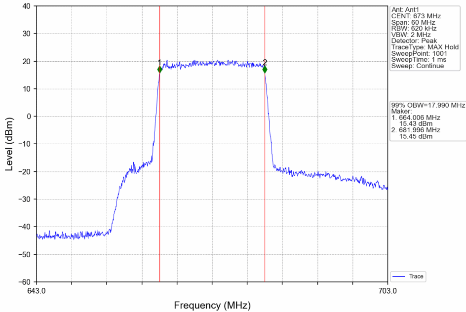
Band71_20MHz_16QAM_LCH_673MHz_RB_100_0_NTNV
