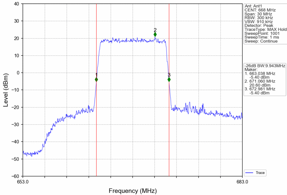
Band71_10MHz_16QAM_LCH_668MHz_RB_50_0_NTNV
