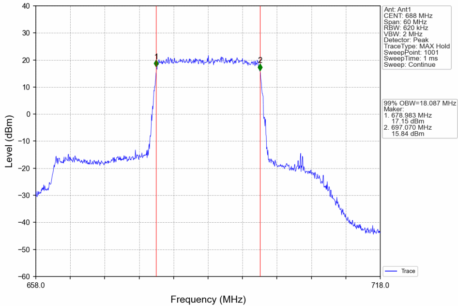
Band71_20MHz_QPSK_HCH_688MHz_RB_100_0_NTNV
