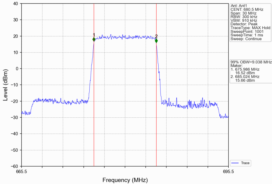
Band71_10MHz_QPSK_MCH_680.5MHz_RB_50_0_NTNV
