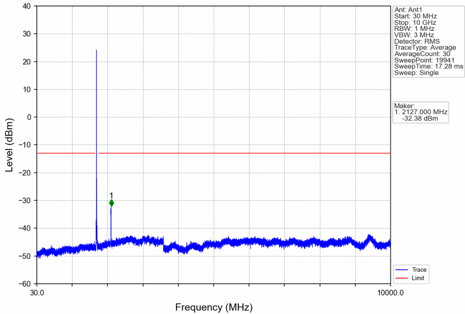
Band66_20MHz_16QAM_LCH_1720MHz_RB_1_0_NTNV
