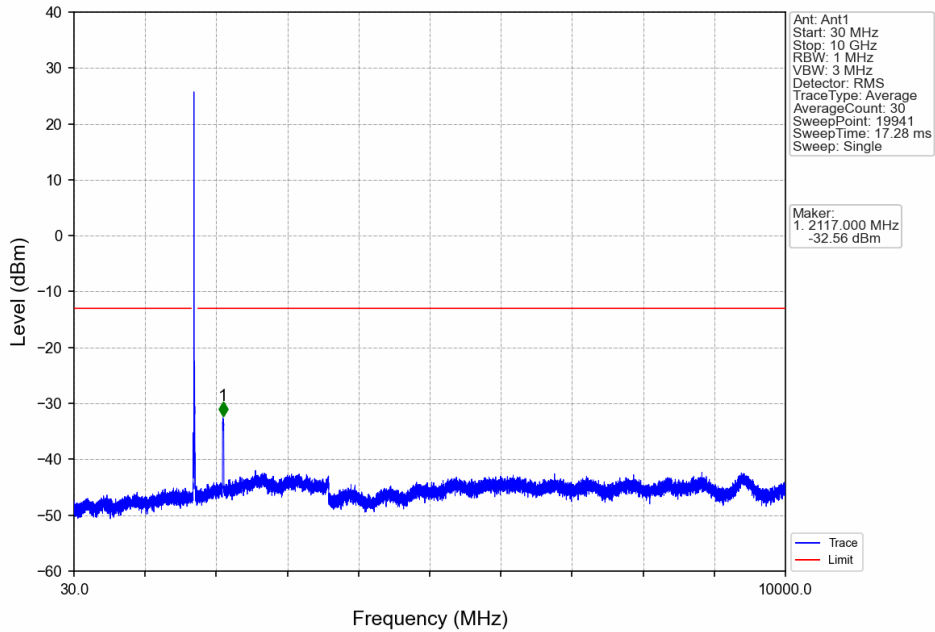
Band66_20MHz_QPSK_LCH_1720MHz_RB_1_0_NTNV
