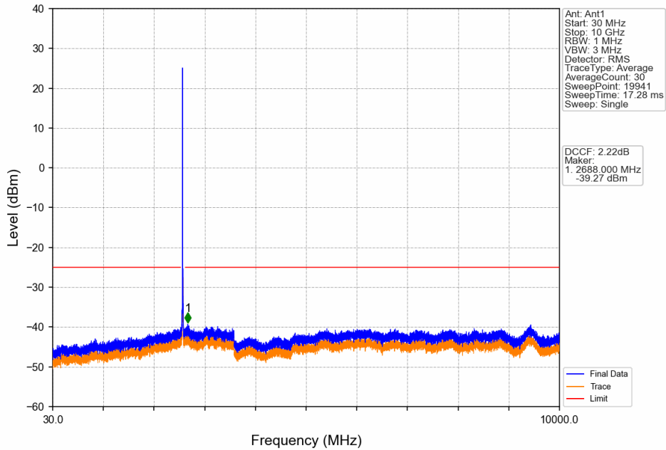
Band41_20MHz_16QAM_MCH_2593MHz_RB_1_0_NTNV
