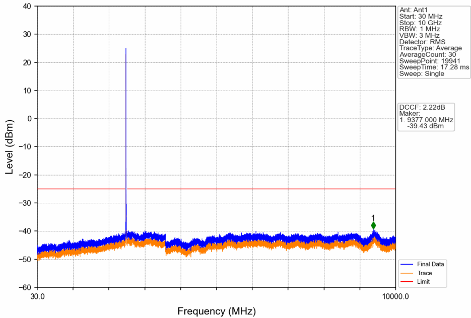
Band41_15MHz_QPSK_LCH_2503.5MHz_RB_1_0_NTNV
