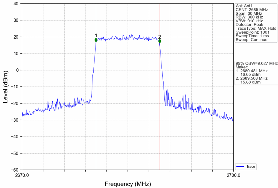
Band41_10MHz_16QAM_HCH_2685MHz_RB_50_0_NTNV
