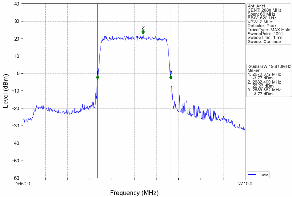
Band41_20MHz_QPSK_HCH_2680MHz_RB_100_0_NTNV
