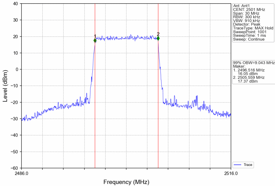
Band41_10MHz_16QAM_LCH_2501MHz_RB_50_0_NTNV
