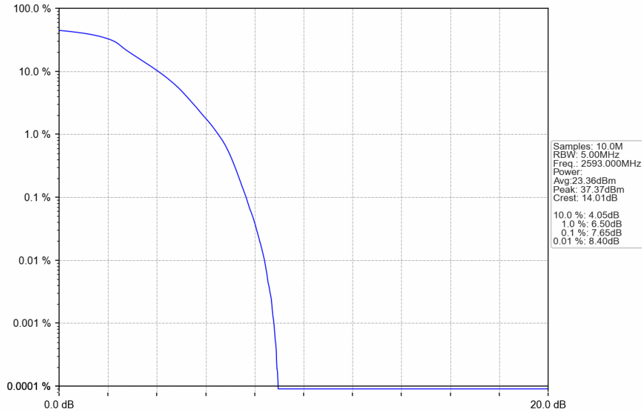
Band41_5MHz_QPSK_MCH_2593MHz_RB_25_0_NTNV
