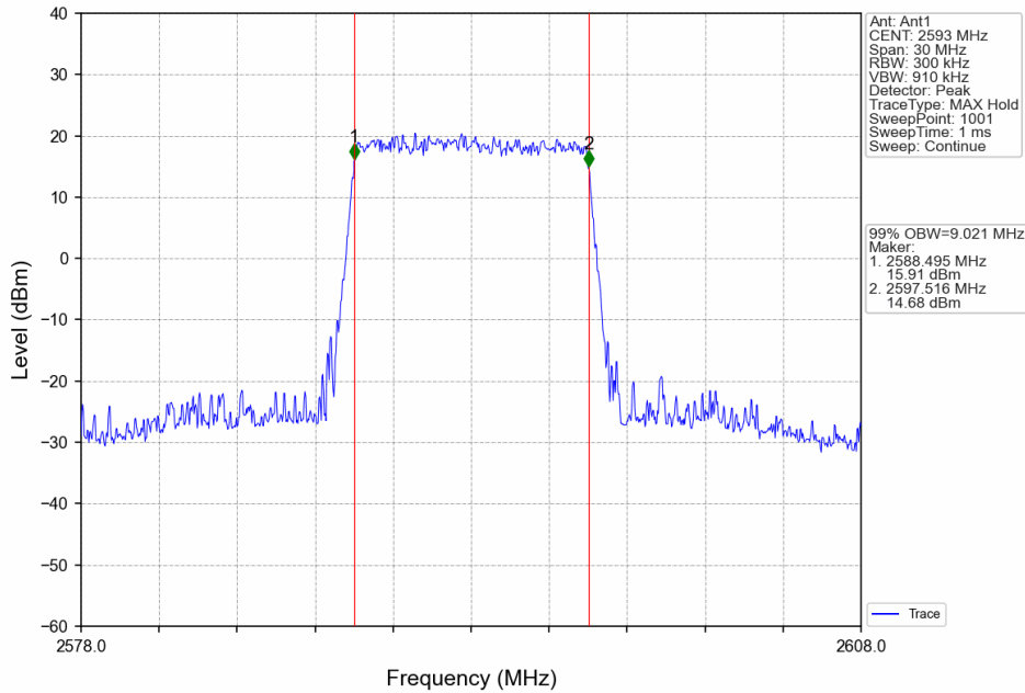
Band41_10MHz_64QAM_MCH_2593MHz_RB_50_0_NTNV
