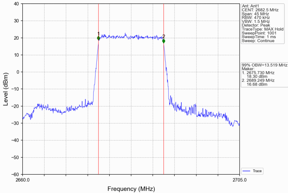
Band41_15MHz_QPSK_HCH_2682.5MHz_RB_75_0_NTNV
