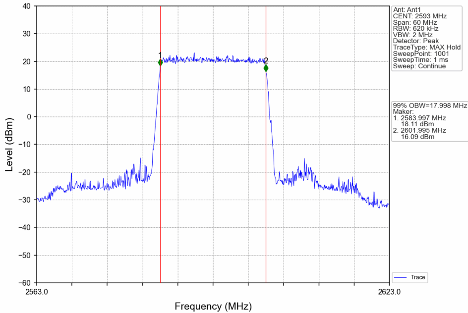
Band41_20MHz_QPSK_MCH_2593MHz_RB_100_0_NTNV
