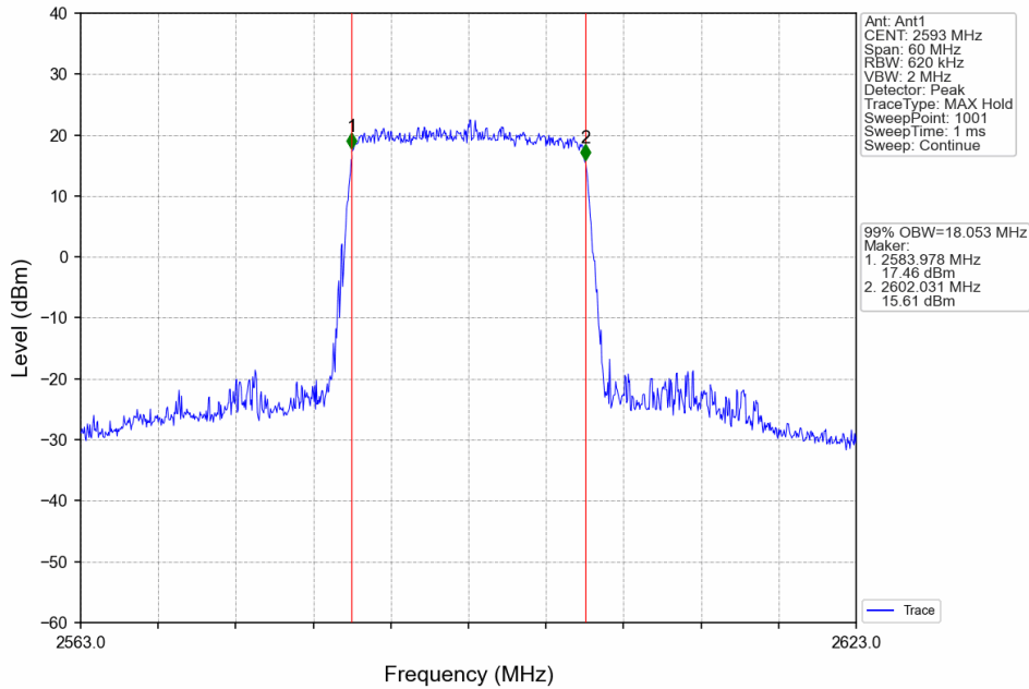
Band41_20MHz_16QAM_MCH_2593MHz_RB_100_0_NTNV
