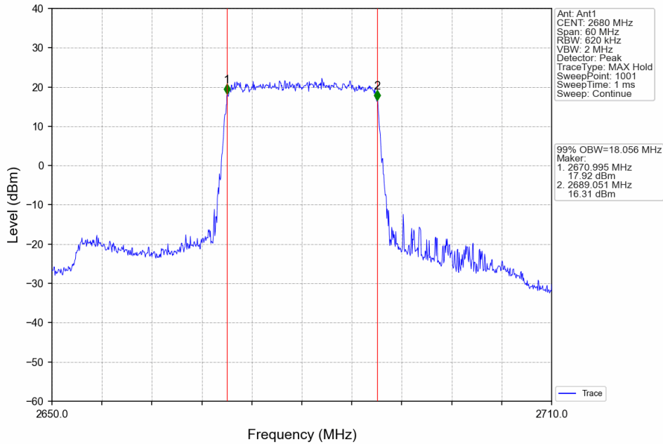
Band41_20MHz_QPSK_HCH_2680MHz_RB_100_0_NTNV
