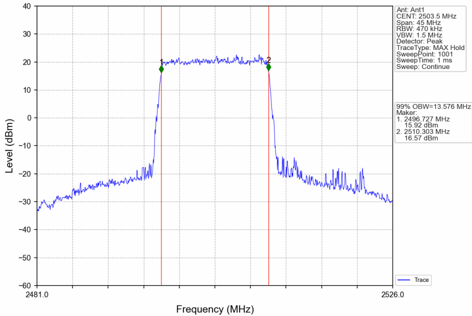
Band41_15MHz_QPSK_LCH_2503.5MHz_RB_75_0_NTNV
