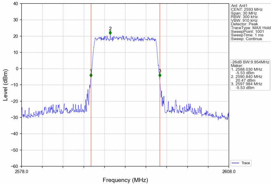
Band41_10MHz_64QAM_MCH_2593MHz_RB_50_0_NTNV
