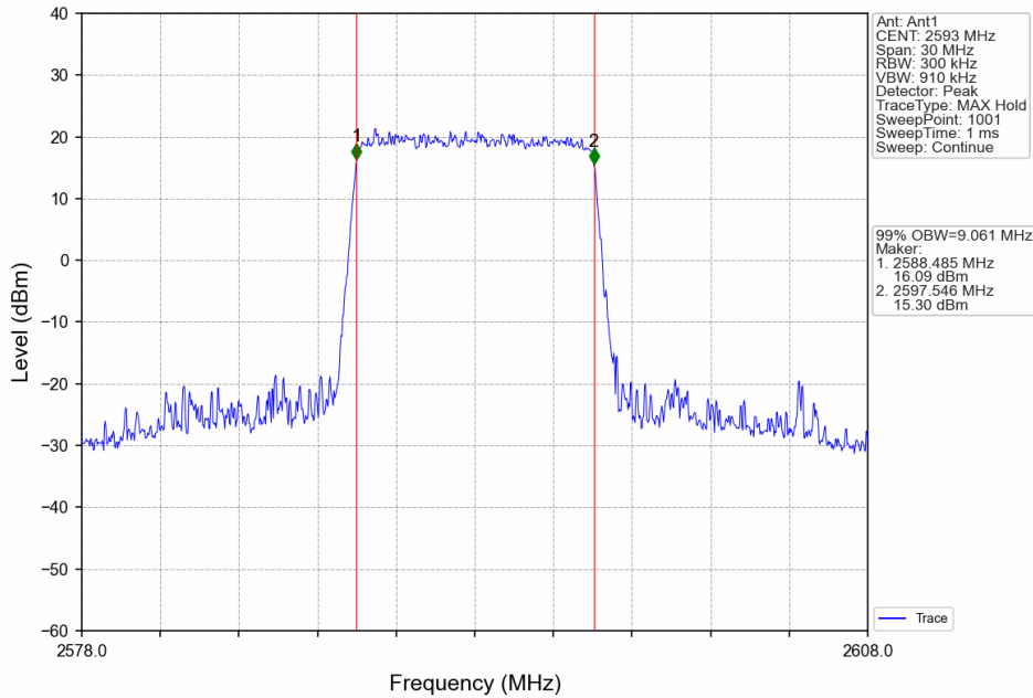
Band41_10MHz_16QAM_MCH_2593MHz_RB_50_0_NTNV
