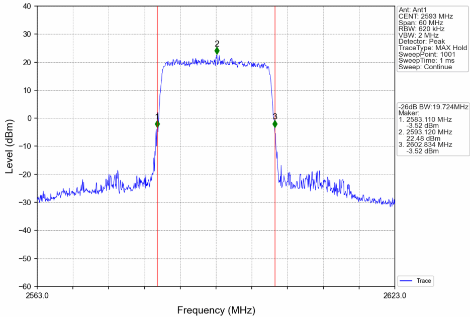
Band41_20MHz_16QAM_MCH_2593MHz_RB_100_0_NTNV
