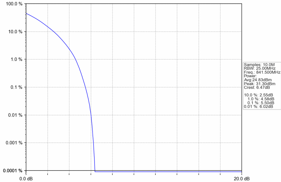
Band26c_15MHz_QPSK_HCH_841.5MHz_RB_75_0_NTNV
