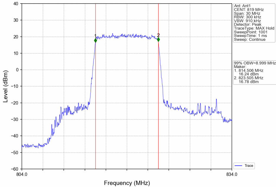
Band26a_10MHz_QPSK_MCH_819MHz_RB_50_0_NTNV
