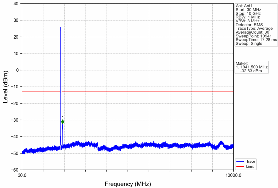
Band25_20MHz_QPSK_LCH_1860MHz_RB_1_0_NTNV
