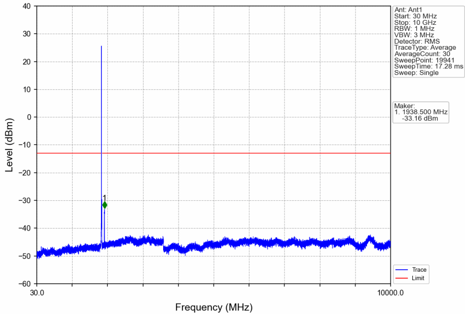
Band25_10MHz_QPSK_LCH_1855MHz_RB_1_0_NTNV
