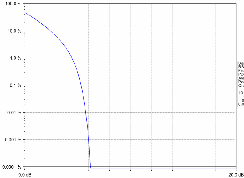
Band25_20MHz_QPSK_HCH_1905MHz_RB_100_0_NTNV
