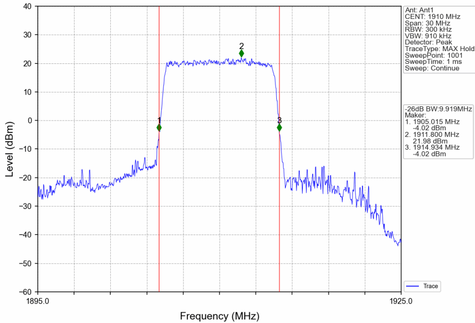
Band25_10MHz_QPSK_HCH_1910MHz_RB_50_0_NTNV
