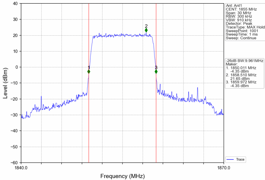
Band25_10MHz_QPSK_LCH_1855MHz_RB_50_0_NTNV
