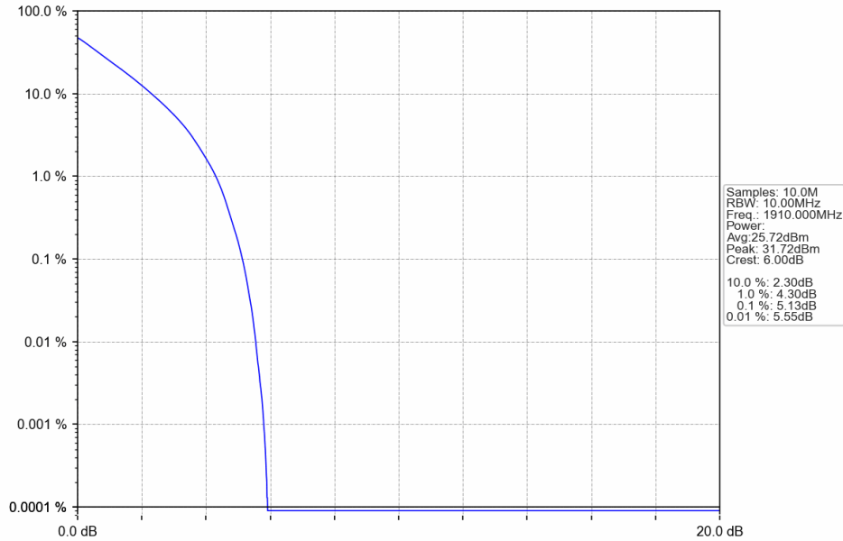
Band25_10MHz_QPSK_HCH_1910MHz_RB_50_0_NTNV
