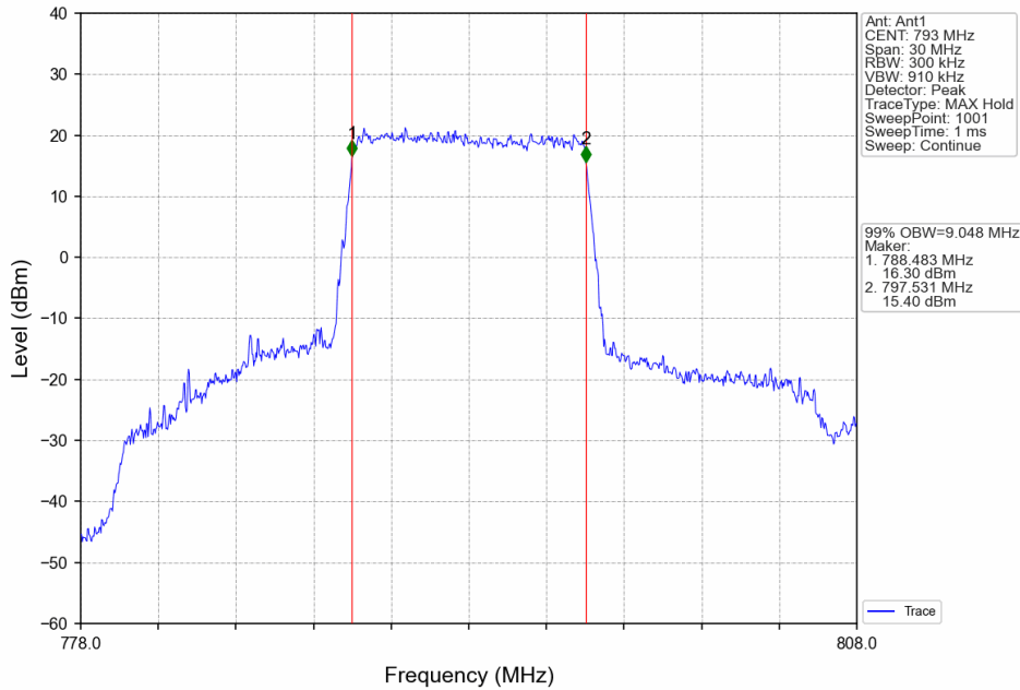
Band14_10MHz_QPSK_MCH_793MHz_RB_50_0_NTNV
