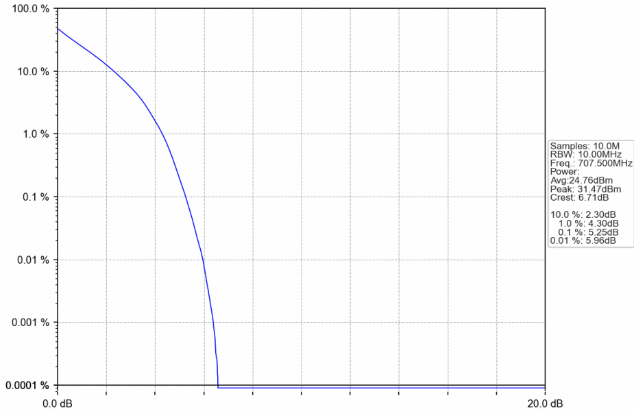
Band12_10MHz_QPSK_MCH_707.5MHz_RB_50_0_NTNV
