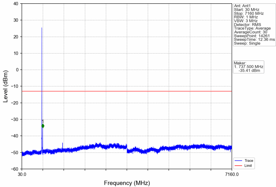
Band12_3MHz_QPSK_MCH_707.5MHz_RB_1_0_NTNV
