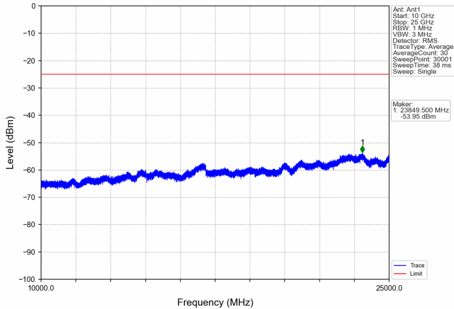
Band7_20MHz_QPSK_MCH_2535MHz_RB_1_0_NTNV
