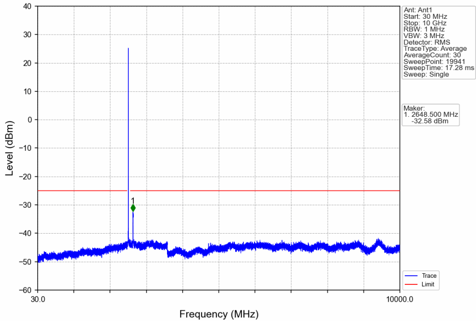
Band7_20MHz_64QAM_MCH_2535MHz_RB_1_0_NTNV
