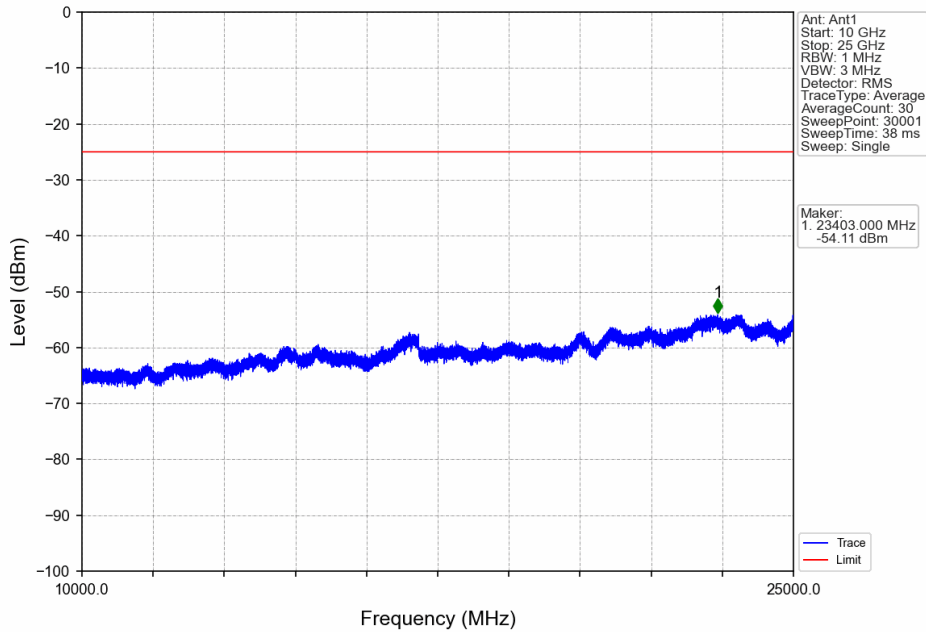
Band7_20MHz_QPSK_HCH_2560MHz_RB_1_0_NTNV
