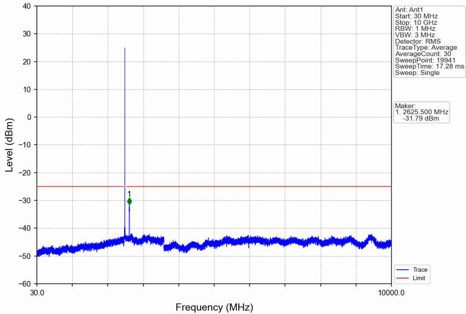
Band7_20MHz_64QAM_LCH_2510MHz_RB_1_0_NTNV
