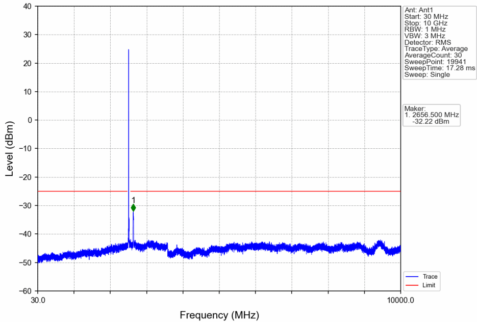
Band7_20MHz_16QAM_MCH_2535MHz_RB_1_0_NTNV
