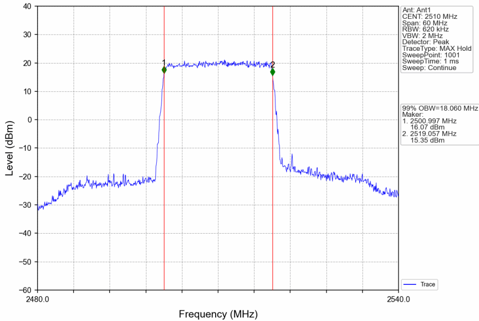
Band7_20MHz_16QAM_LCH_2510MHz_RB_100_0_NTNV
