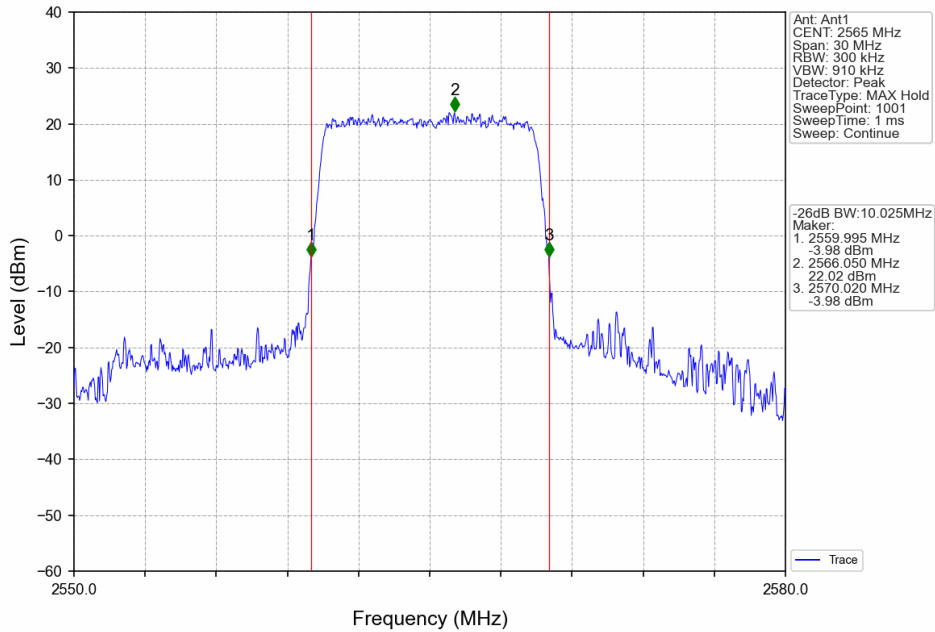
Band7_10MHz_QPSK_HCH_2565MHz_RB_50_0_NTNV
