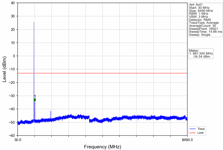
Band5_10MHz_QPSK_HCH_844MHz_RB_1_0_NTNV
