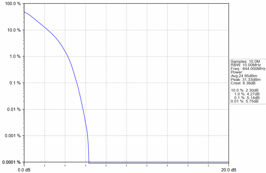
Band5_10MHz_QPSK_HCH_844MHz_RB_50_0_NTNV
