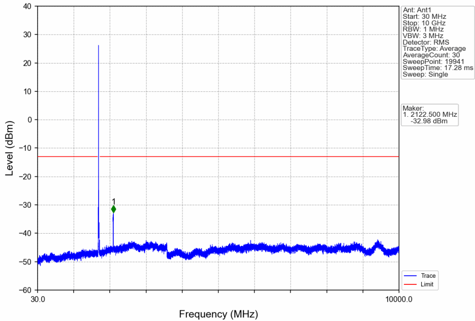
Band4_15MHz_QPSK_LCH_1717.5MHz_RB_1_0_NTNV
