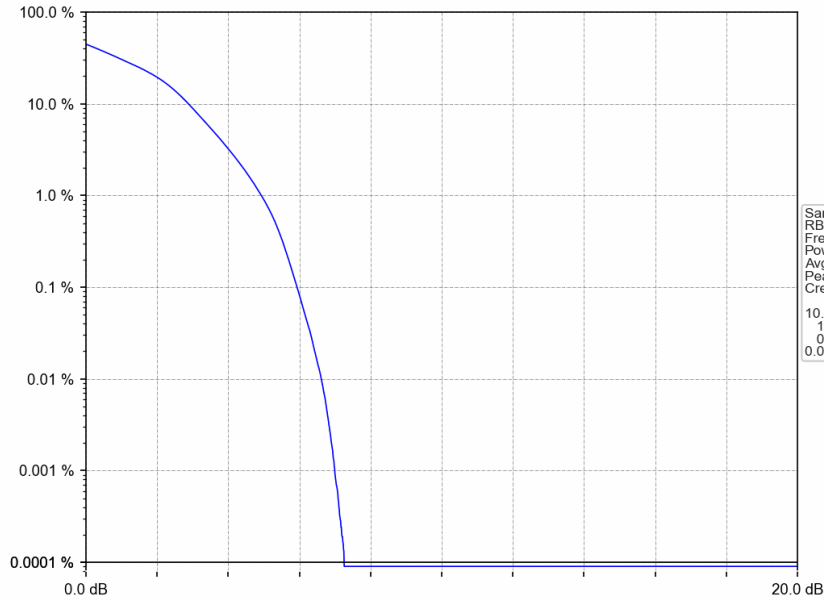
Band4_20MHz_16QAM_LCH_1720MHz_RB_100_0_NTNV
