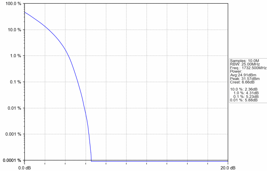
Band4_20MHz_QPSK_MCH_1732.5MHz_RB_100_0_NTNV
