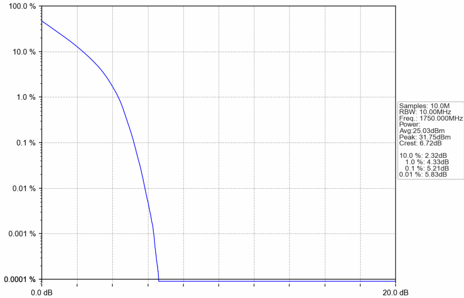
Band4_10MHz_QPSK_HCH_1750MHz_RB_50_0_NTNV
