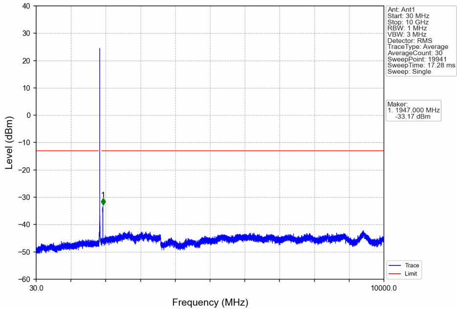
Band2_20MHz_16QAM_LCH_1860MHz_RB_1_0_NTNV
