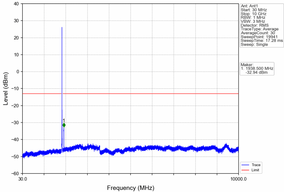
Band2_15MHz_QPSK_LCH_1857.5MHz_RB_1_0_NTNV
