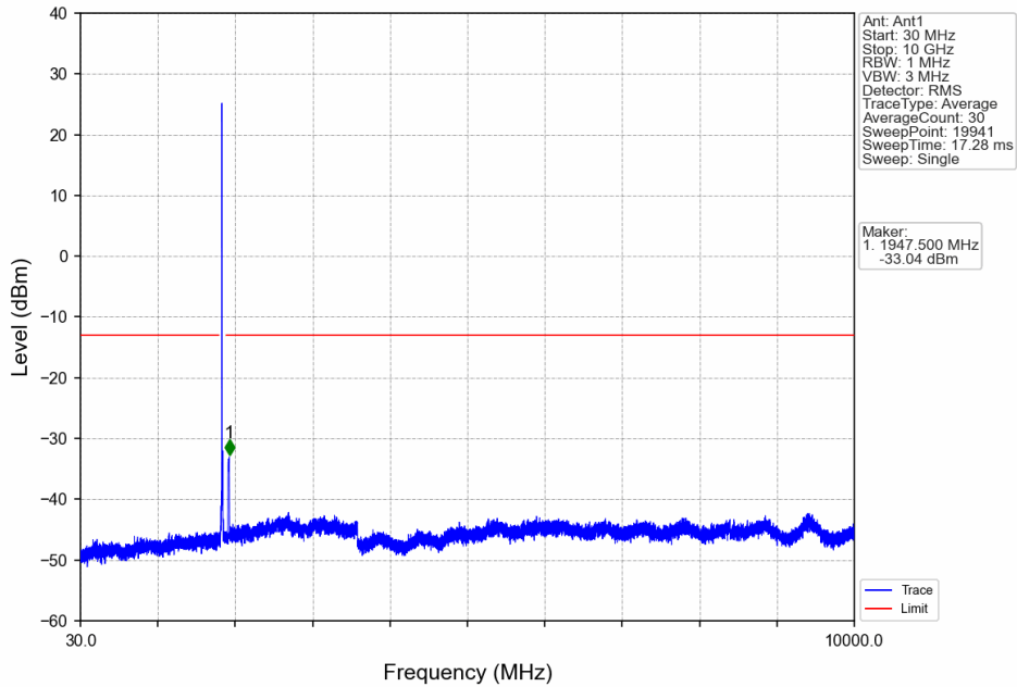
Band2_20MHz_QPSK_LCH_1860MHz_RB_1_0_NTNV
