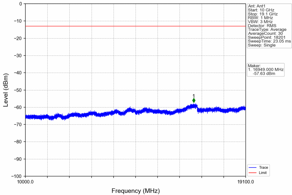
Band2_20MHz_QPSK_LCH_1860MHz_RB_1_0_NTNV
