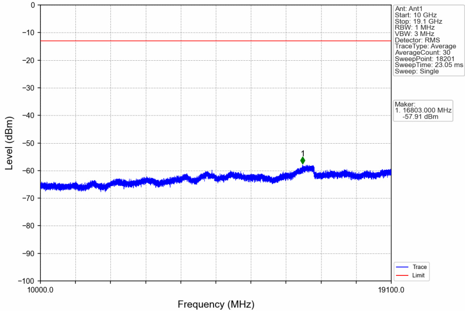
Band2_20MHz_16QAM_MCH_1880MHz_RB_1_0_NTNV
