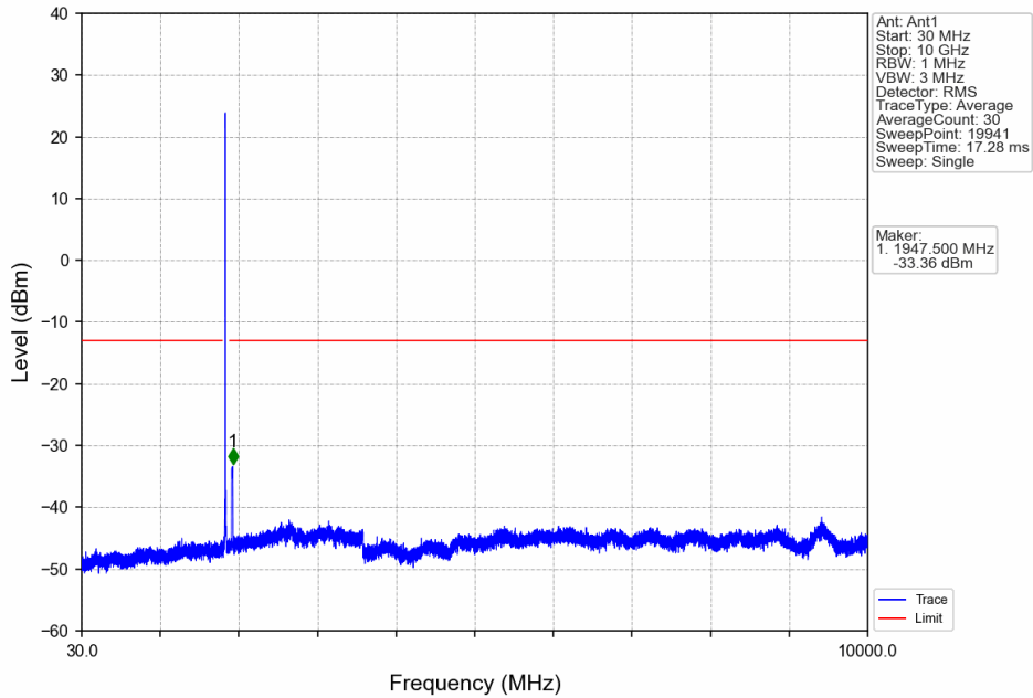
Band2_20MHz_64QAM_LCH_1860MHz_RB_1_0_NTNV
