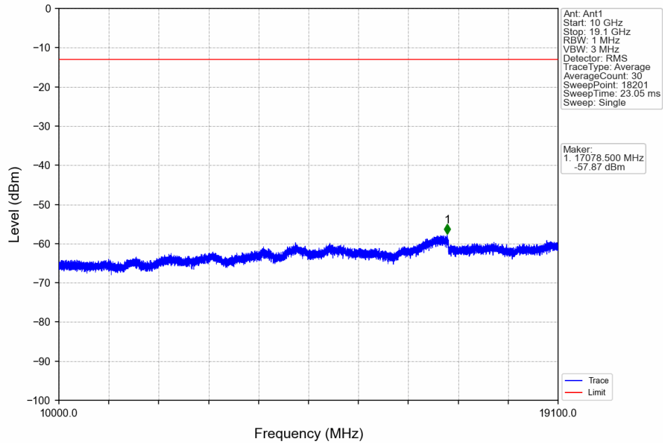
Band2_3MHz_16QAM_MCH_1880MHz_RB_1_0_NTNV
