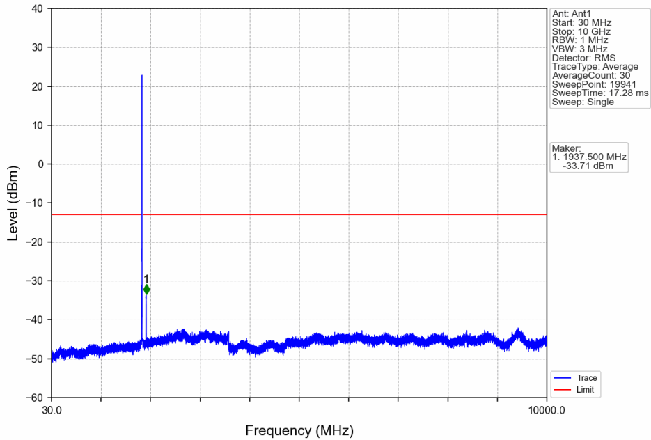
Band2_10MHz_64QAM_LCH_1855MHz_RB_1_0_NTNV
