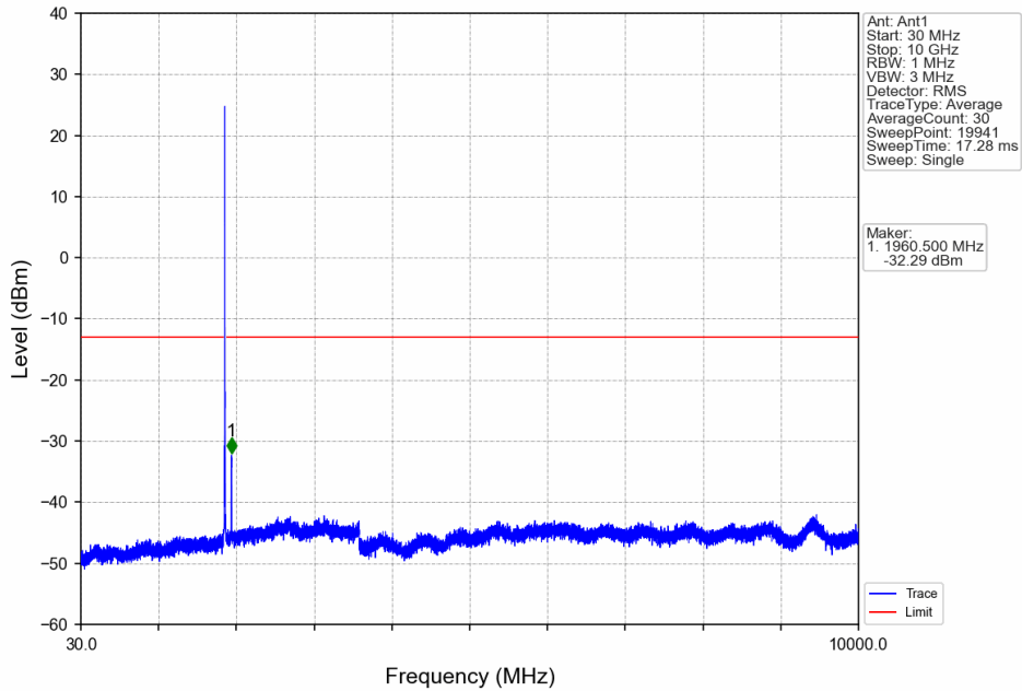
Band2_10MHz_16QAM_MCH_1880MHz_RB_1_0_NTNV
