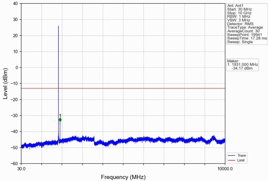
Band2_3MHz_QPSK_LCH_1851.5MHz_RB_1_0_NTNV
