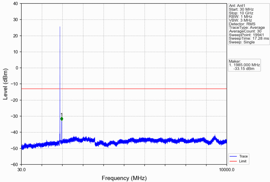
Band2_10MHz_16QAM_HCH_1905MHz_RB_1_0_NTNV
