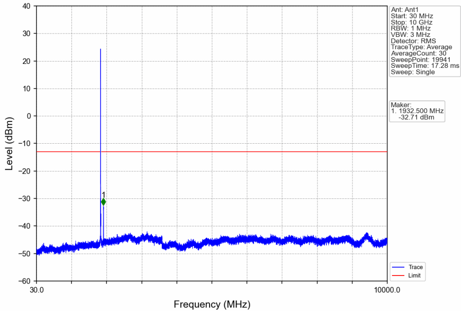
Band2_10MHz_16QAM_LCH_1855MHz_RB_1_0_NTNV
