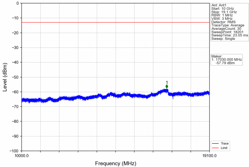
Band2_10MHz_64QAM_LCH_1855MHz_RB_1_0_NTNV
