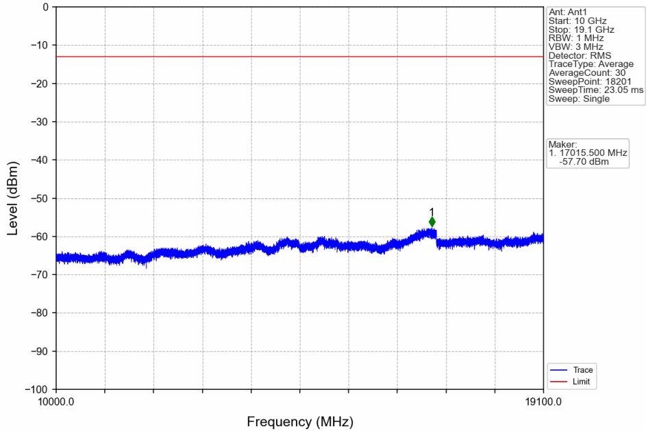
Band2_10MHz_QPSK_LCH_1855MHz_RB_1_0_NTNV
