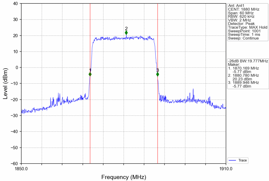
Band2_20MHz_64QAM_MCH_1880MHz_RB_100_0_NTNV
