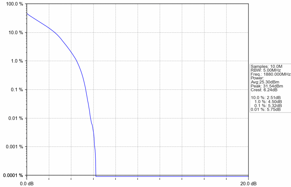
Band2_3MHz_QPSK_MCH_1880MHz_RB_15_0_NTNV
