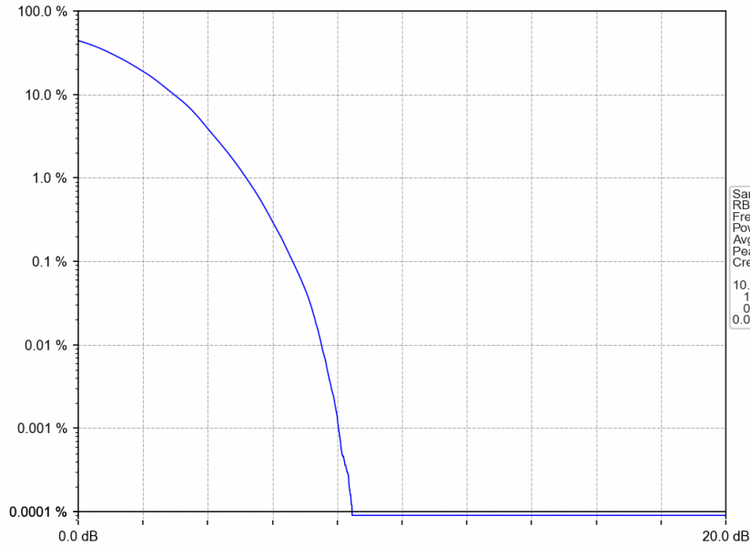
Band2_20MHz_64QAM_MCH_1880MHz_RB_100_0_NTNV
