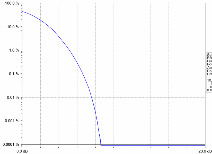
Band2_20MHz_64QAM_LCH_1860MHz_RB_100_0_NTNV
