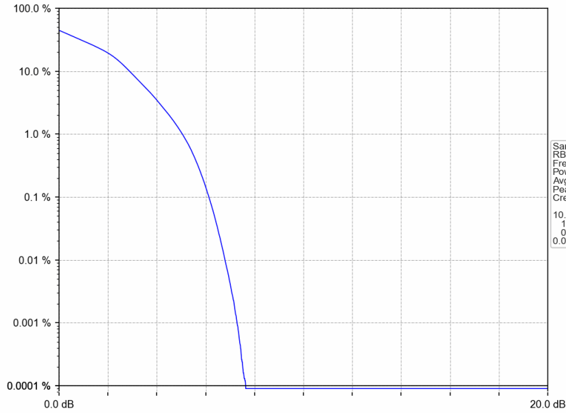
Band2_20MHz_16QAM_HCH_1900MHz_RB_100_0_NTNV
