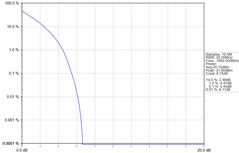
Band2_20MHz_QPSK_HCH_1900MHz_RB_100_0_NTNV
