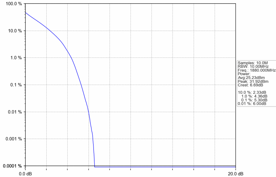
Band2_10MHz_QPSK_MCH_1880MHz_RB_50_0_NTNV
