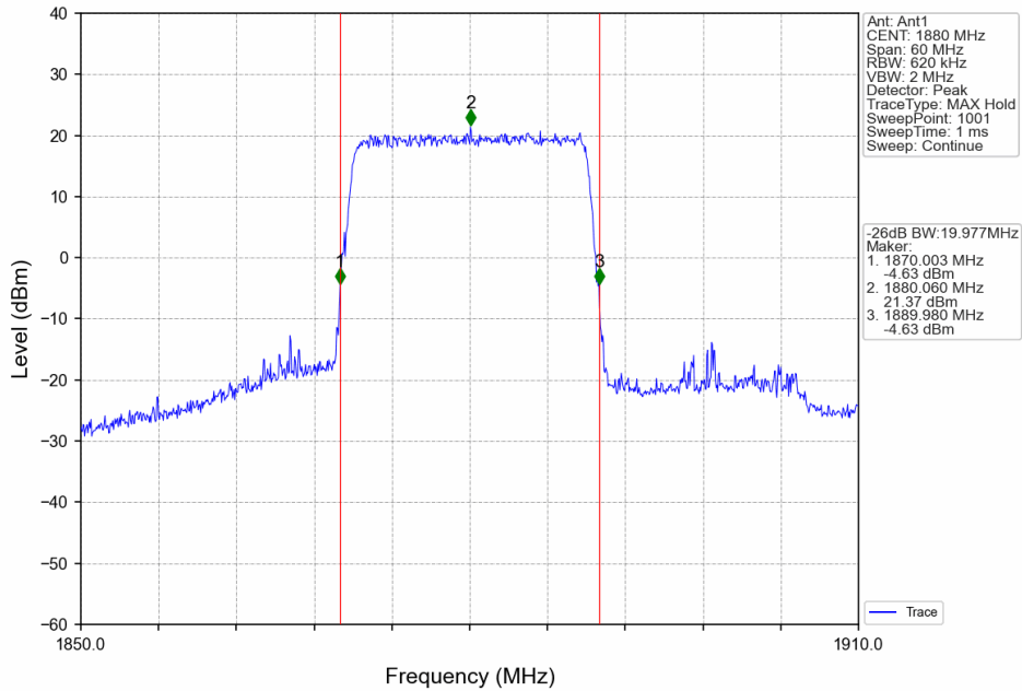
Band2_20MHz_16QAM_MCH_1880MHz_RB_100_0_NTNV
