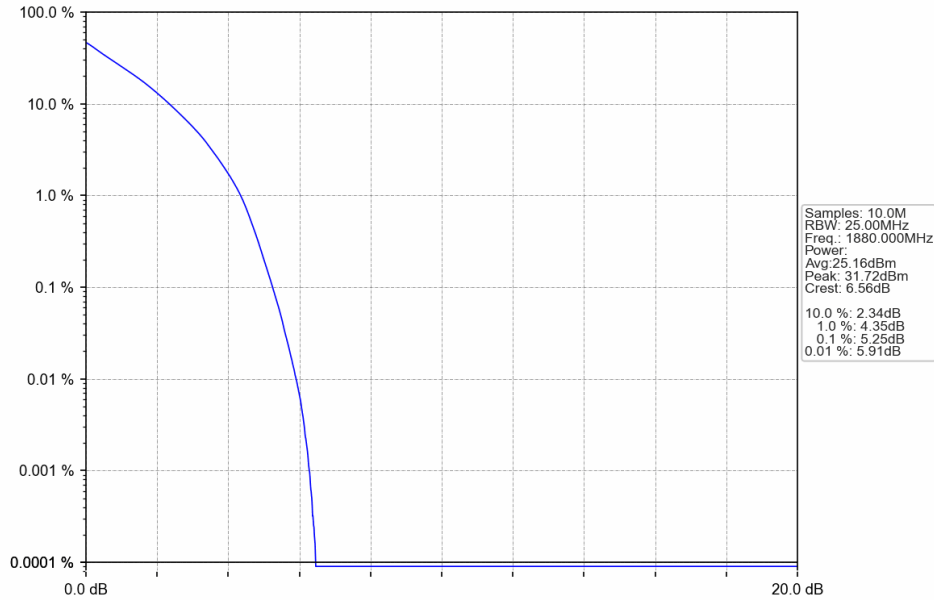
Band2_20MHz_QPSK_MCH_1880MHz_RB_100_0_NTNV
