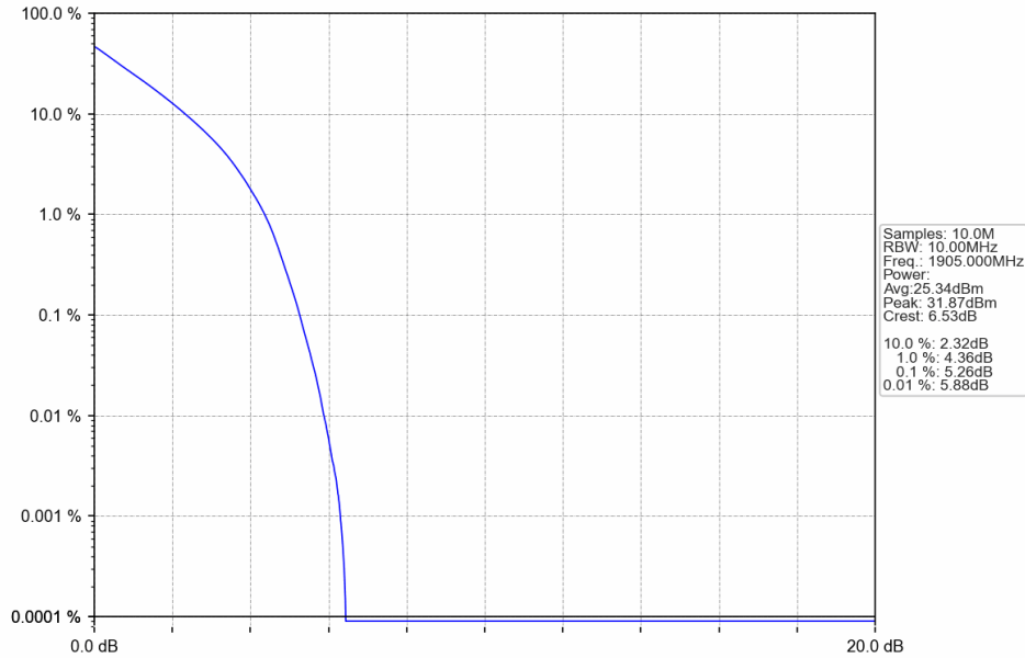
Band2_10MHz_QPSK_HCH_1905MHz_RB_50_0_NTNV
