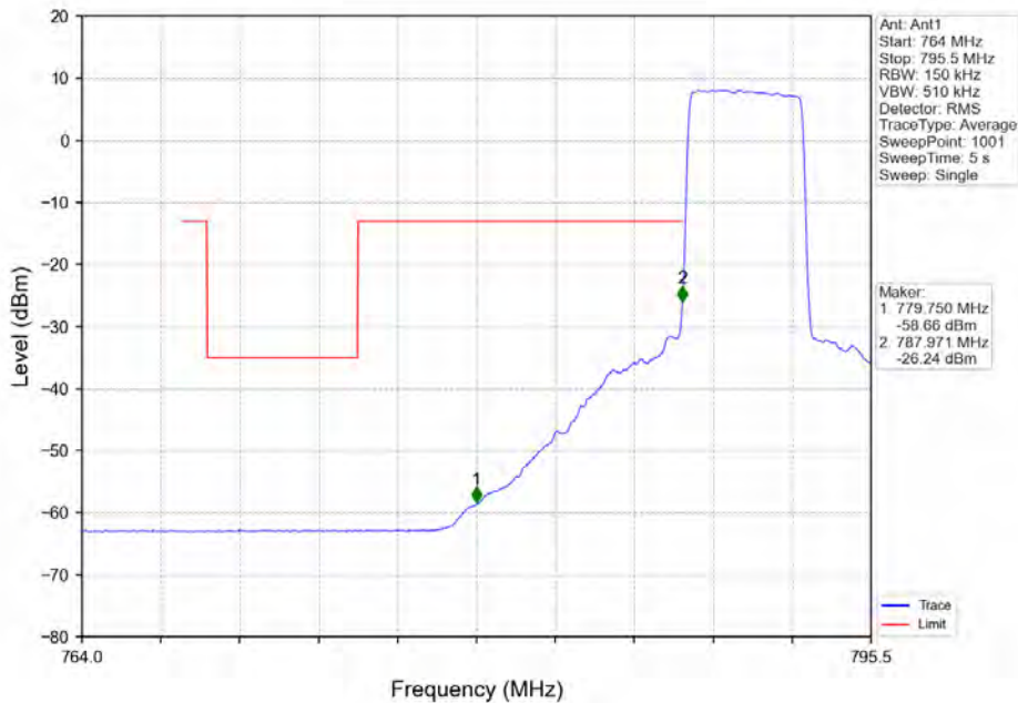
Band 14 5MHz 16QAM LCH 790.5MHz RB 25 0 NTV
