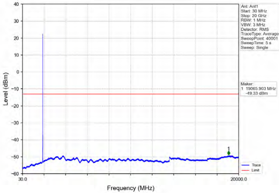
Band 2 10MHz QPSK HCH 1905MHz RB 1 49 NTN
