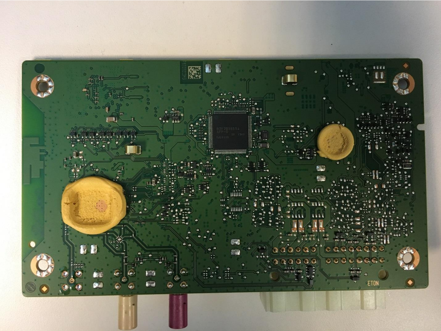
Fig. 2. FB40-ND1 Main pcb side 1.
