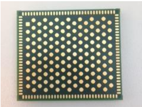
Fig. 3. CUW module bottom view
