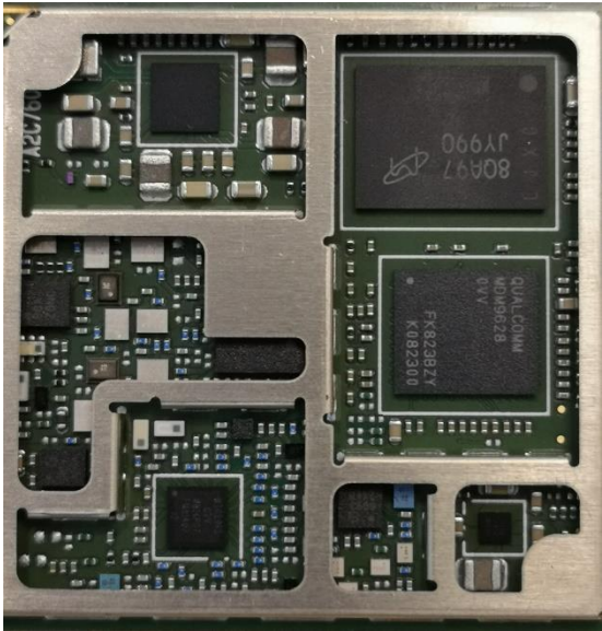
Fig. 1 BL28RW-001 module top view
