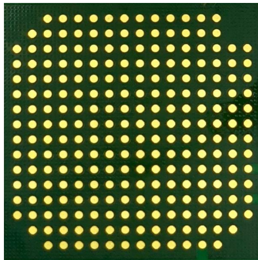
Fig. 4. BL28NA-003 module bottom view
