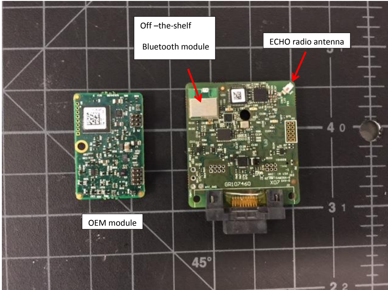
PCBAs
