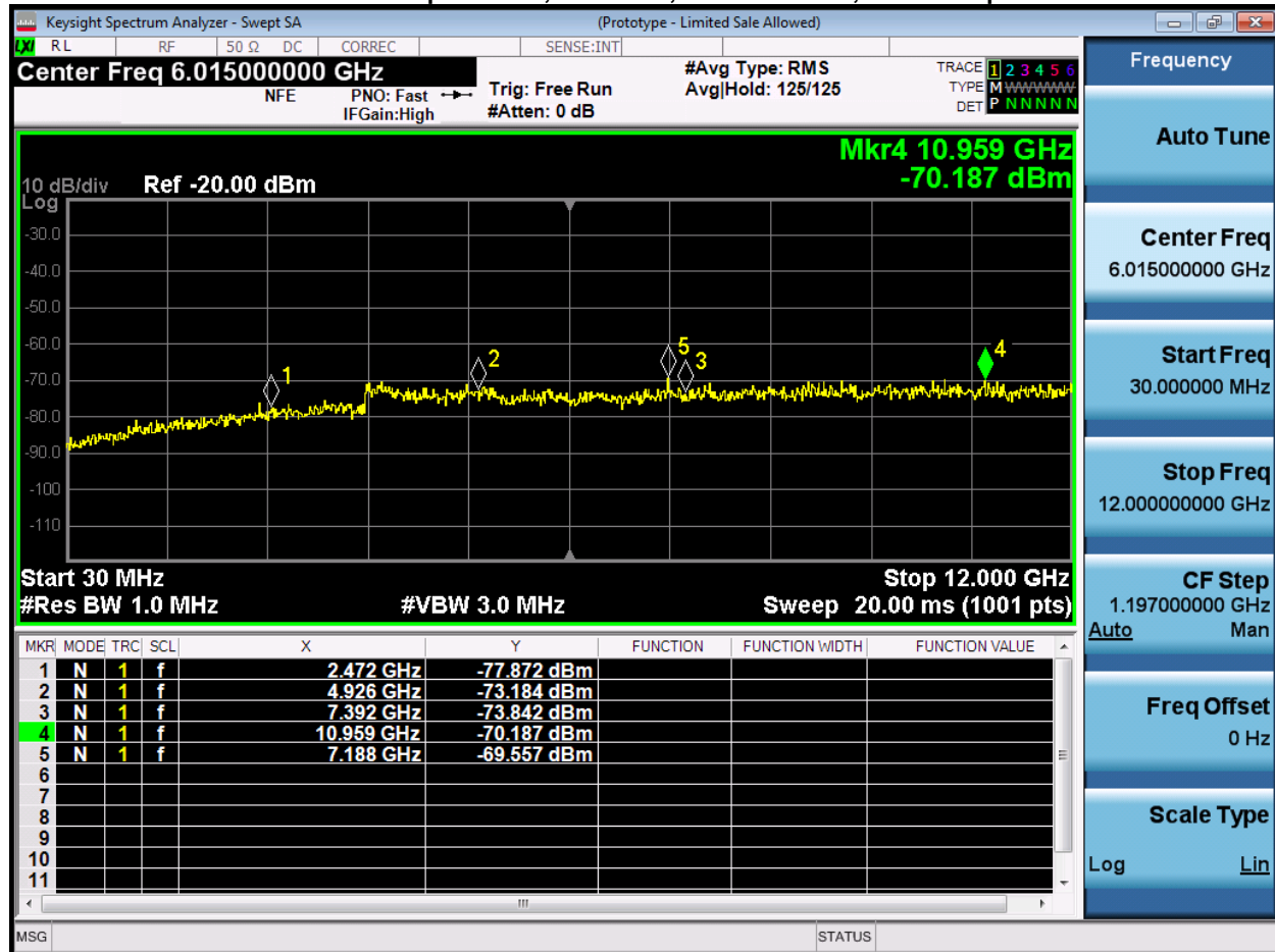
Antenna A
