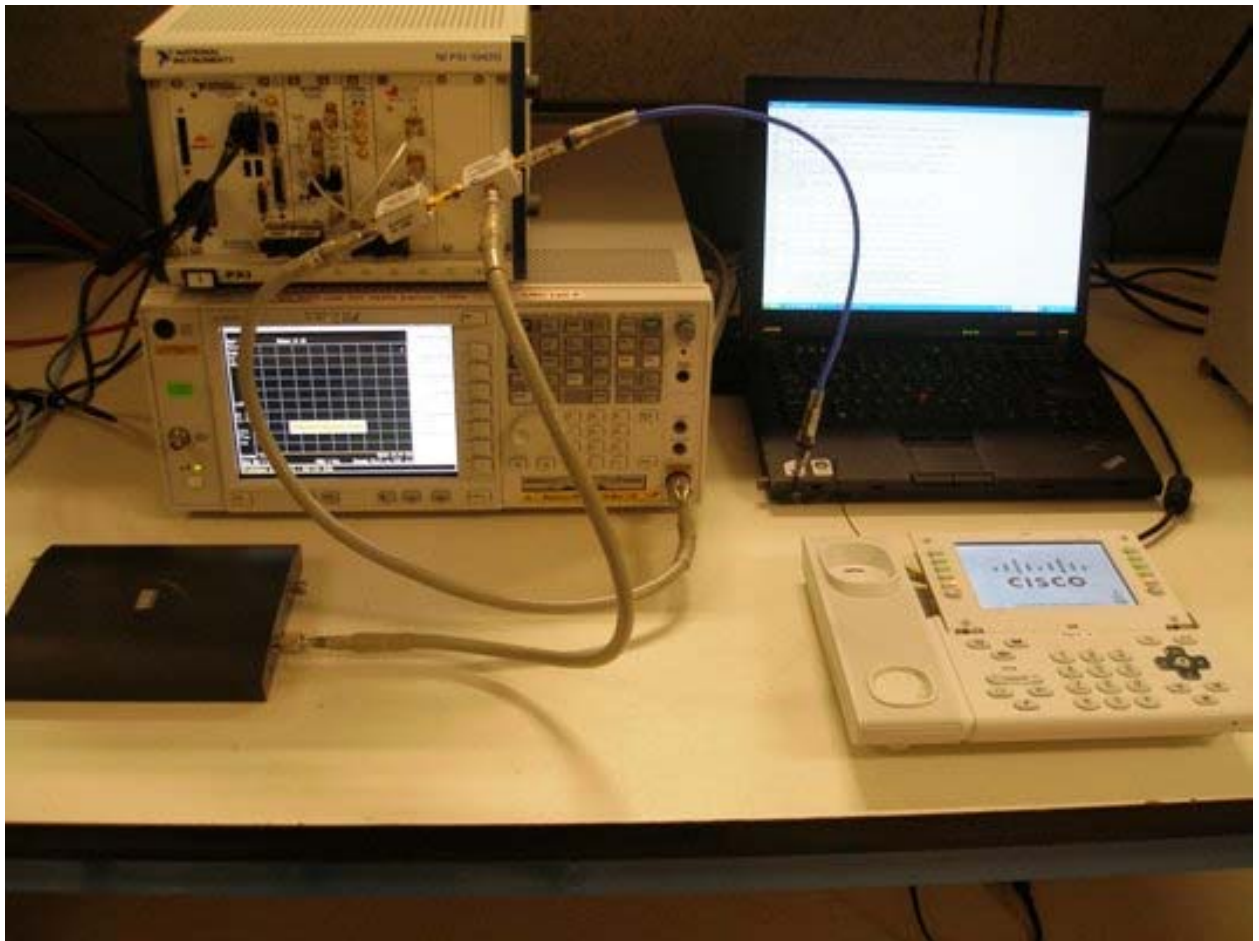
DFS Setup: UUT
