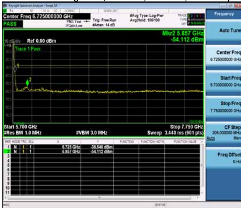
Antenna A
