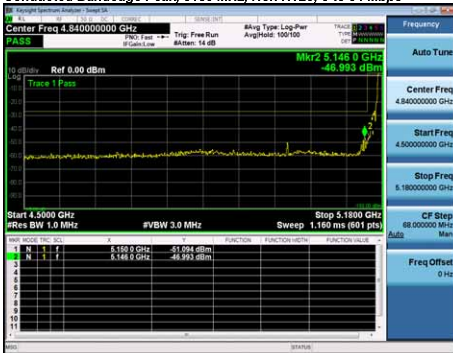
Antenna A
