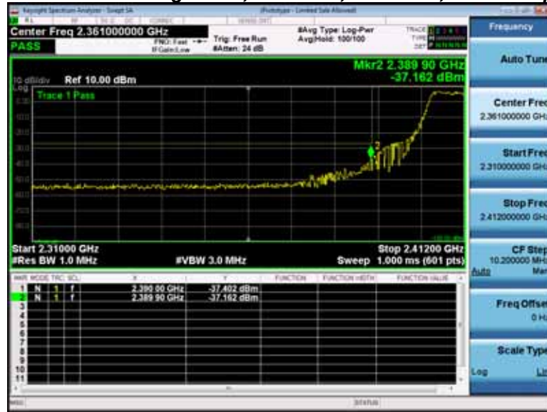
Antenna A
